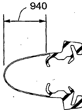
Fig. 94C SECTION A-A
