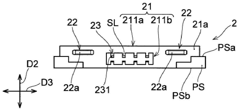
도면9
