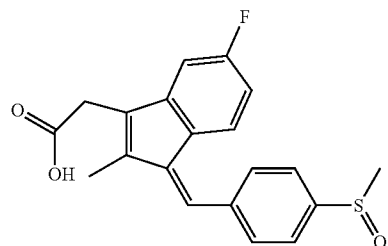
Sulindac
