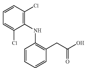
Diclofenac
