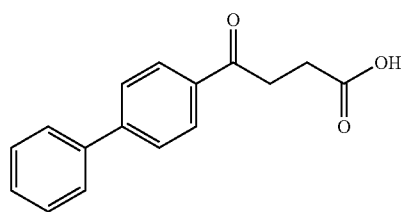
Fenbufen
