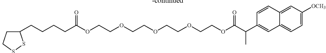
ALA-TEG-Npx
