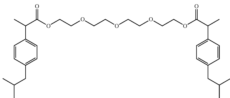
Tetraethylene glycol(ibuprofen) 2
