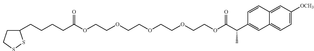
( \alpha -Lipoic acid)-tetraethylene glycol(naproxen)
