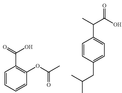
Aspirin
