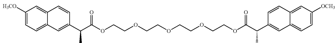
Tetraethylene glycol(naproxen) 2
