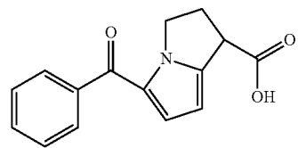
Ketorolac
