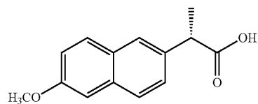
Naproxen
