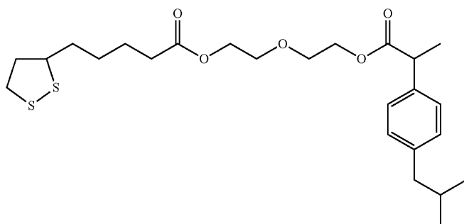
( \alpha -Lipoic acid)-diethylene glycol(ibuprofen)
