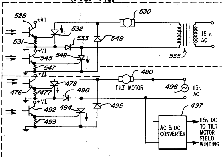
TILT MOTOR SWITCHING CKT.
