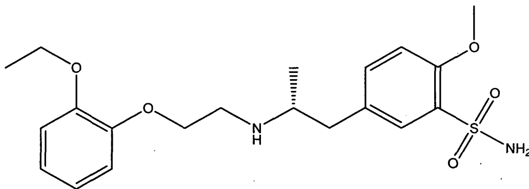
tamsulosin
