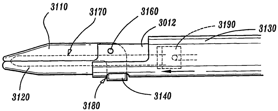
FIG. 39D
