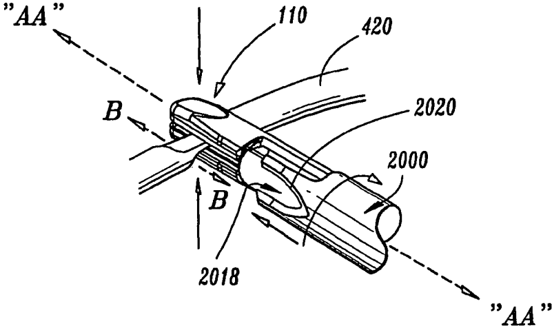
FIG. 37B
