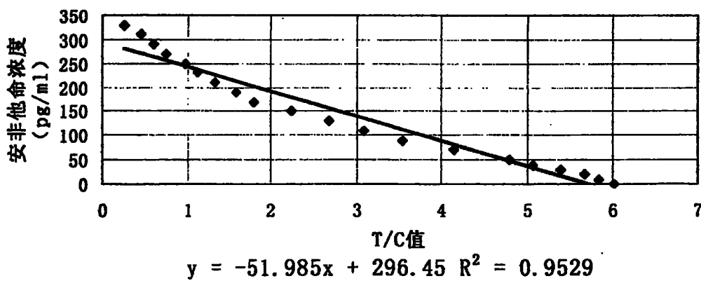
安非他命检测标准工作曲线
