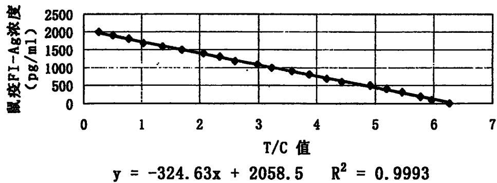
鼠疫FI-Ag检测标准工作曲线
