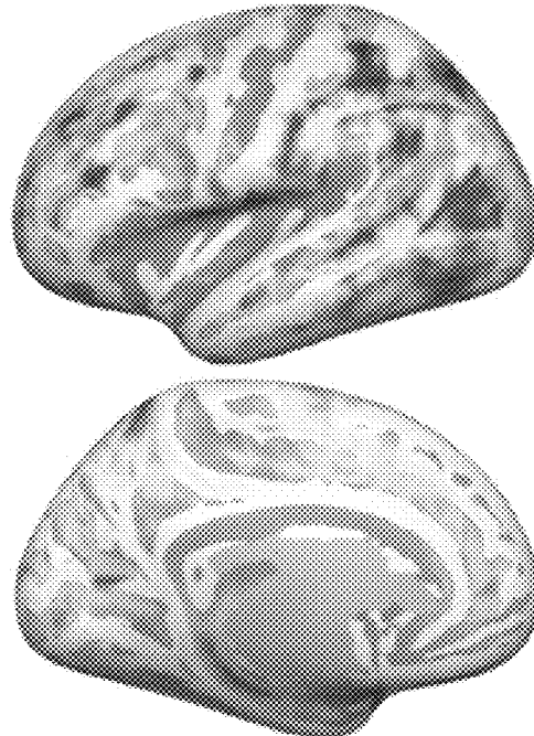
Sulcal Depth Variability
