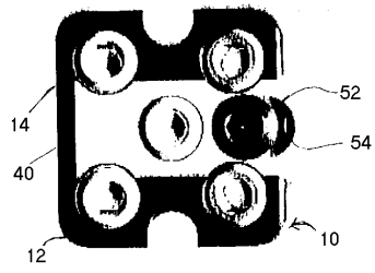
잠금되지 않은 위치의 슬라이더 플레이트
