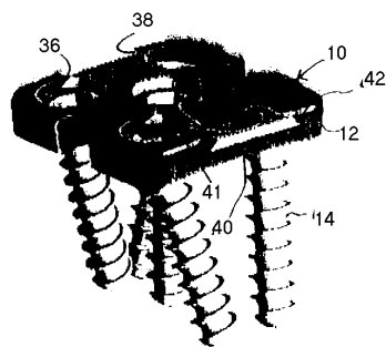
잠금되지 않은 위치의 슬라이더 플레이트
