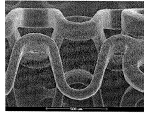
03-05-156-26 EVA-BMA / 3.3%シロリムス (Sirolimus) の基部被膜と、 BMAの上部被膜とにより、被覆されている SEMモードにおけるSEM顕微鏡写真 (100倍)
