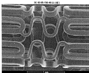
03-05-156-40 EVA-BMA / 3.3%シロリムス (Sirolimus) の基部被膜により、被覆されている SEMモードにおけるSEM顕微鏡写真 (100倍)
