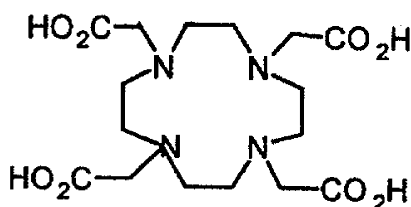
16 (DOTA)
