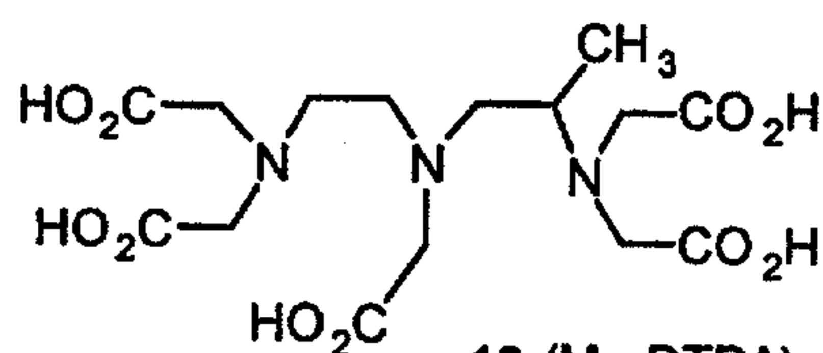
13 (Me-DTPA)
