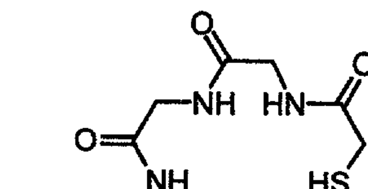
10 (N 3 S)
