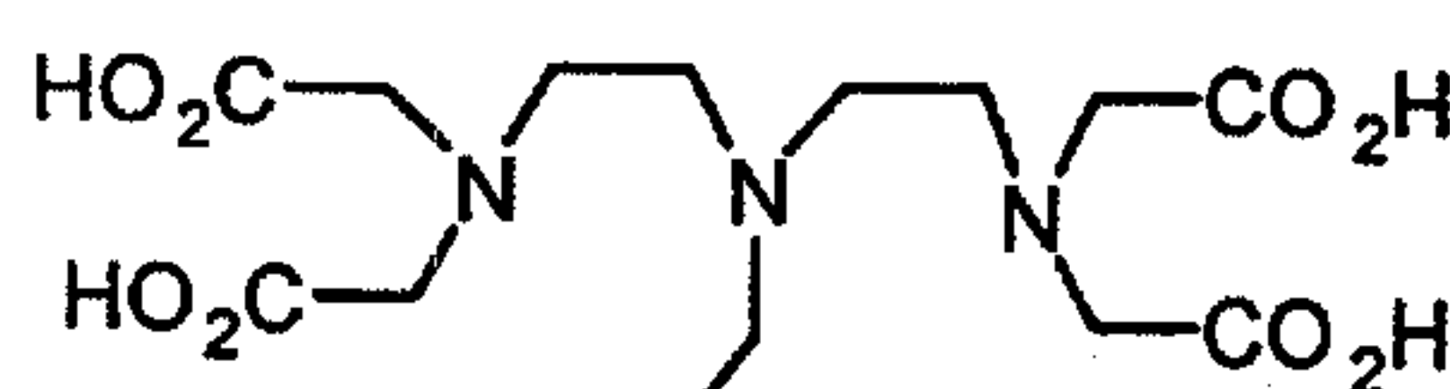
12 (DTPA)
