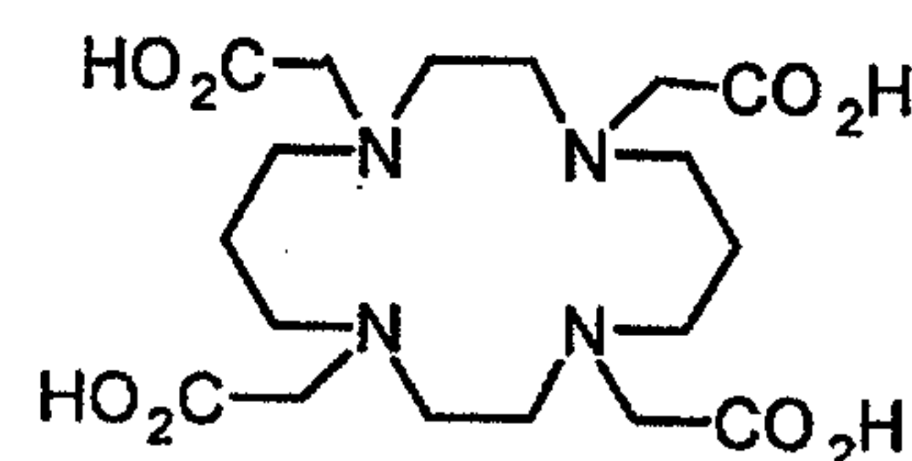
17 (TETA)
