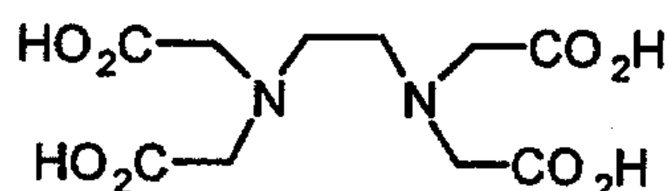
11 (EDTA)
