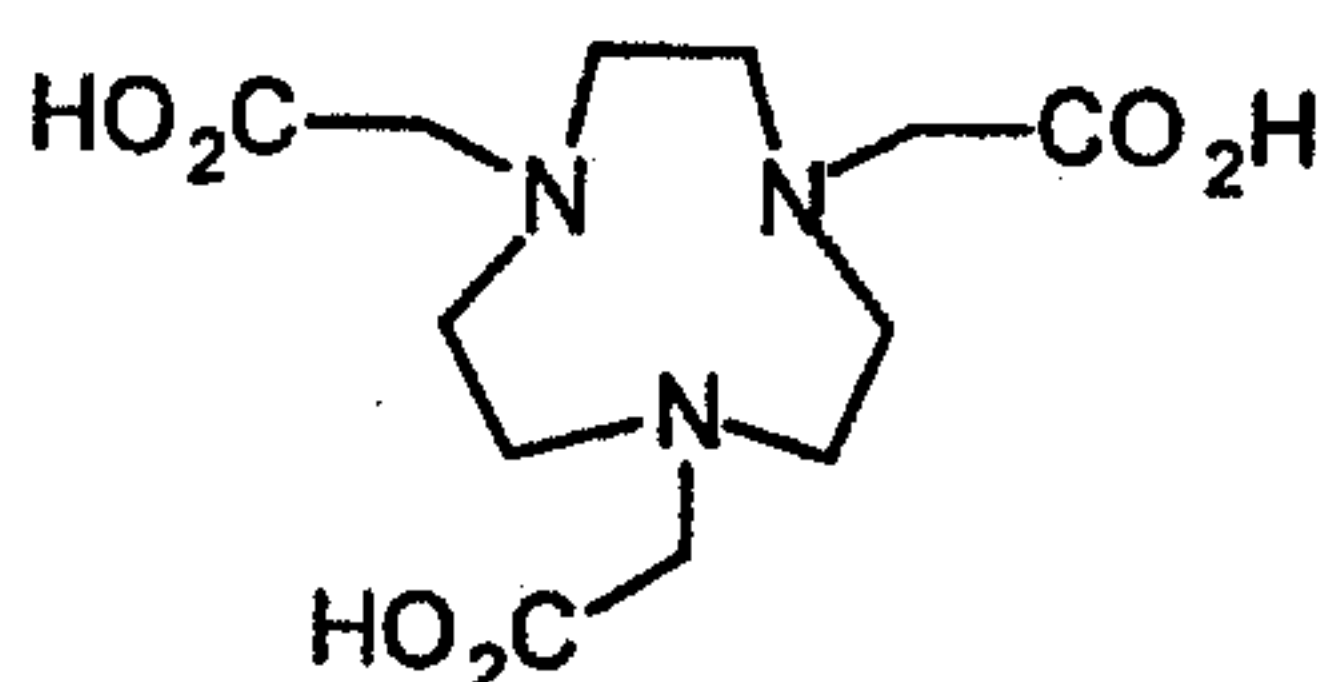
15 (NOTA)
