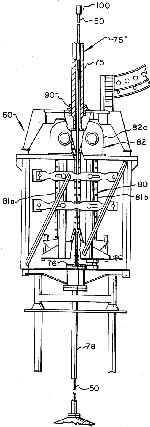
FIG. 15B
