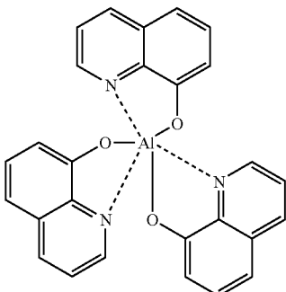
Alq
