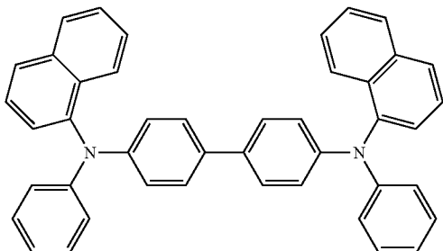
\alpha -NPD
