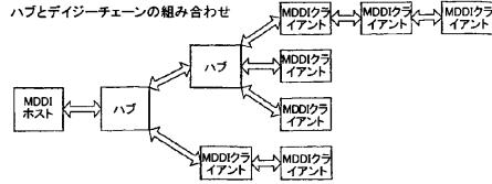
図 99 ハブとデイジーチェーンの組み合わせ
