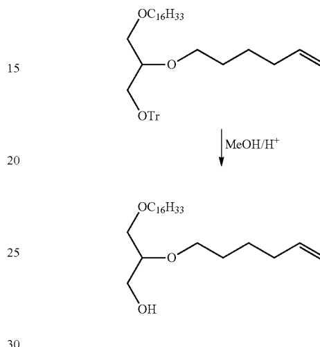
Scheme VI
