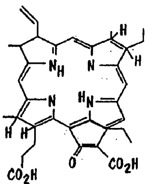
BACTACIOPHAOPHORBIDE
