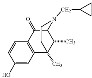
Ethylketocyclazocine (EKC)
