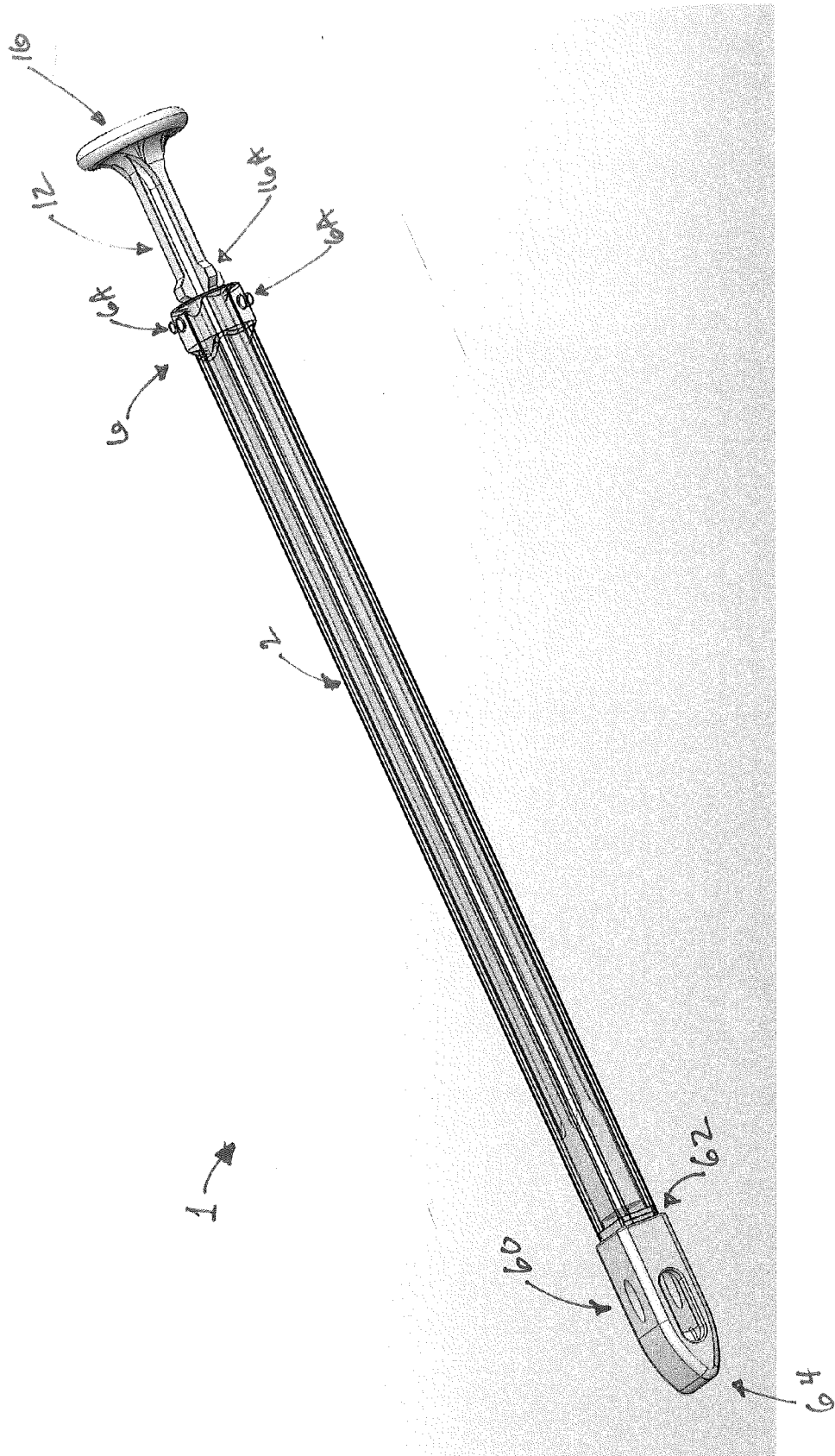
FIG. 37
