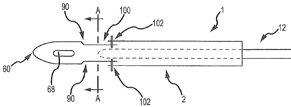
FIG.17A
