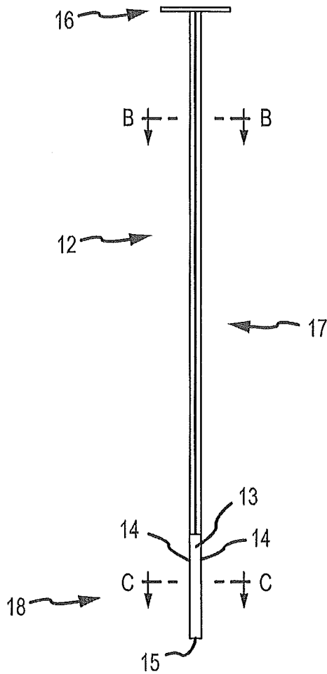
FIG.29
