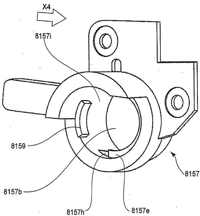
도면59
