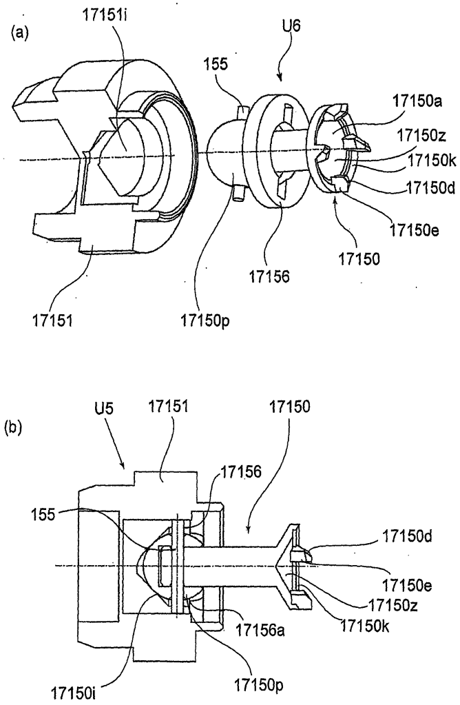
도면107
