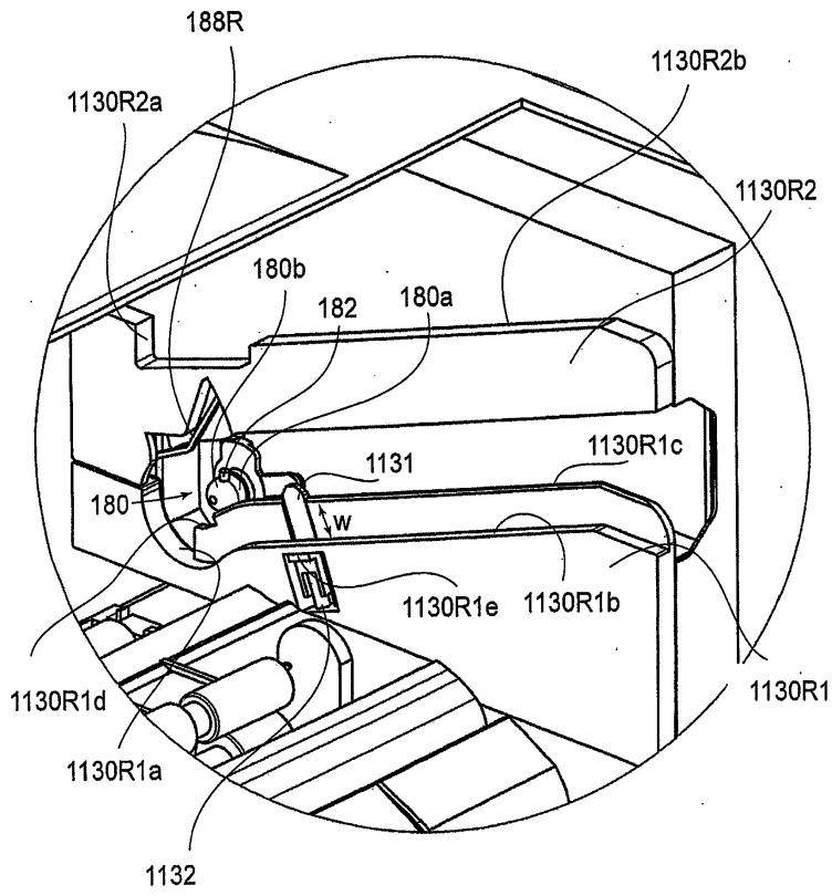
도면75
