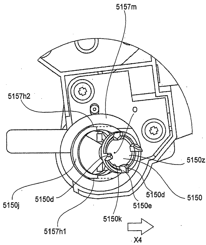
도면55
