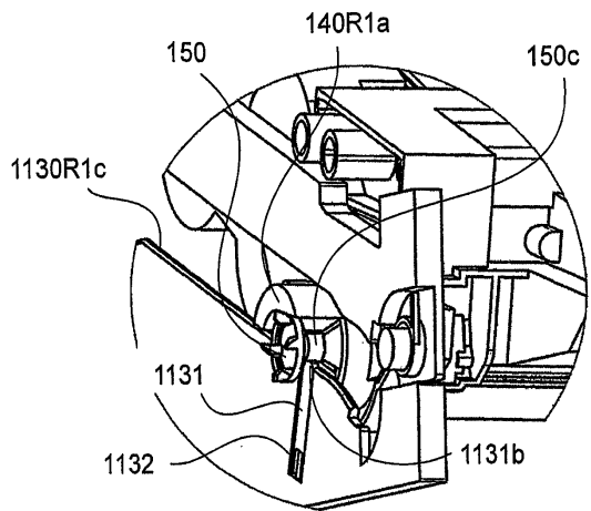
도면79
