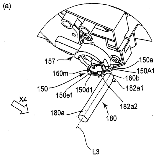
도면21
