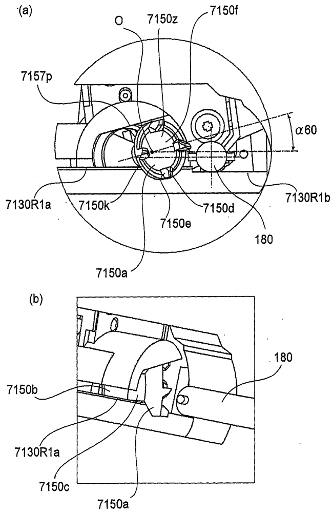
도면72
