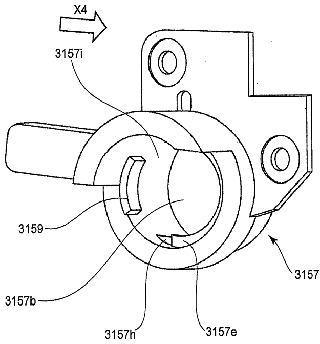
도면47
