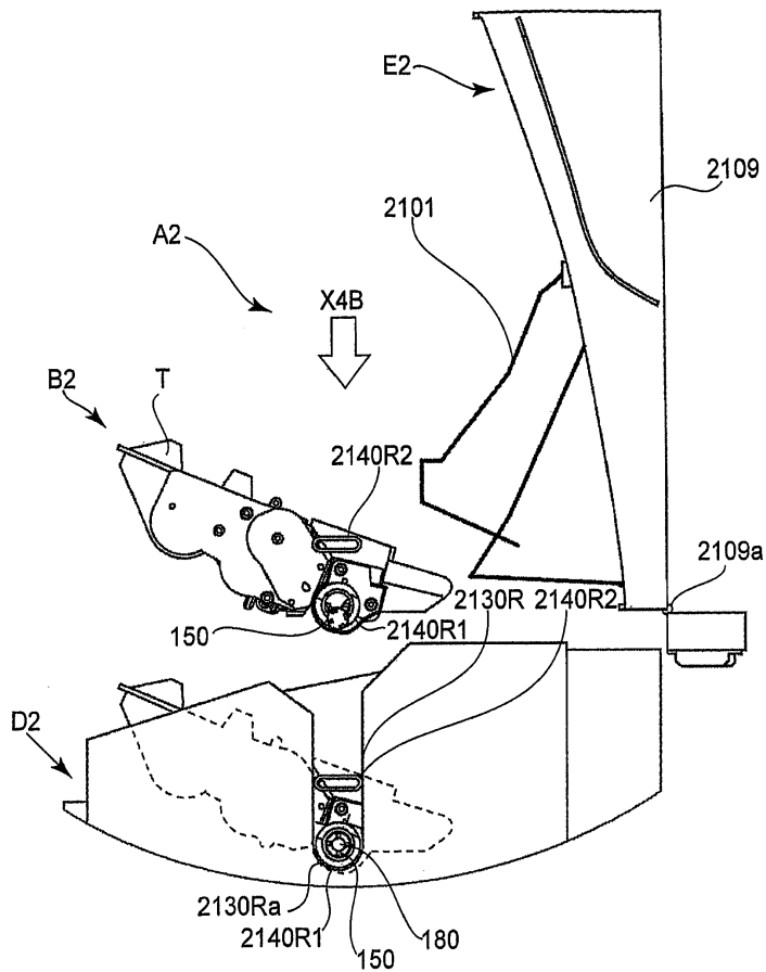
도면45
