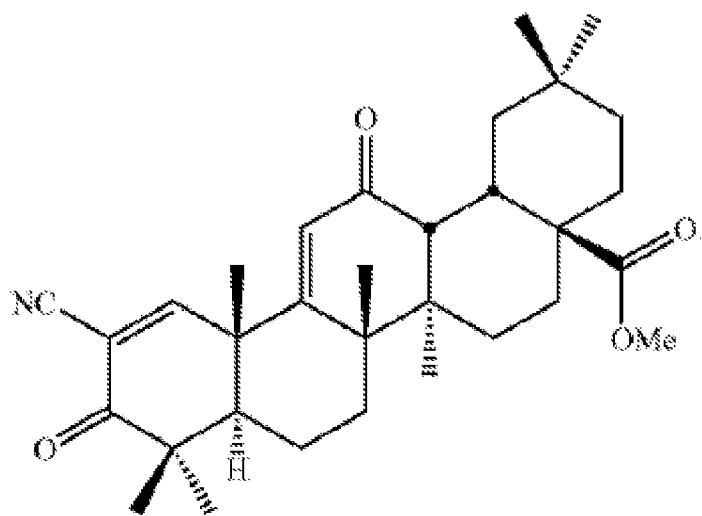
(CDDO-Me, RTA 402)
