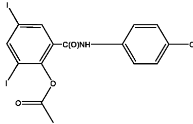
clioxanide
