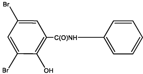
dibromosalalan
