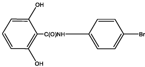
resorantel
