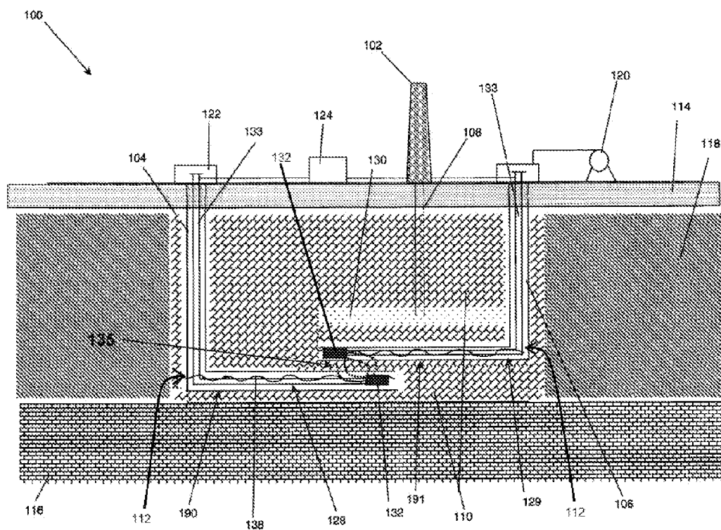
FIG. 1E
