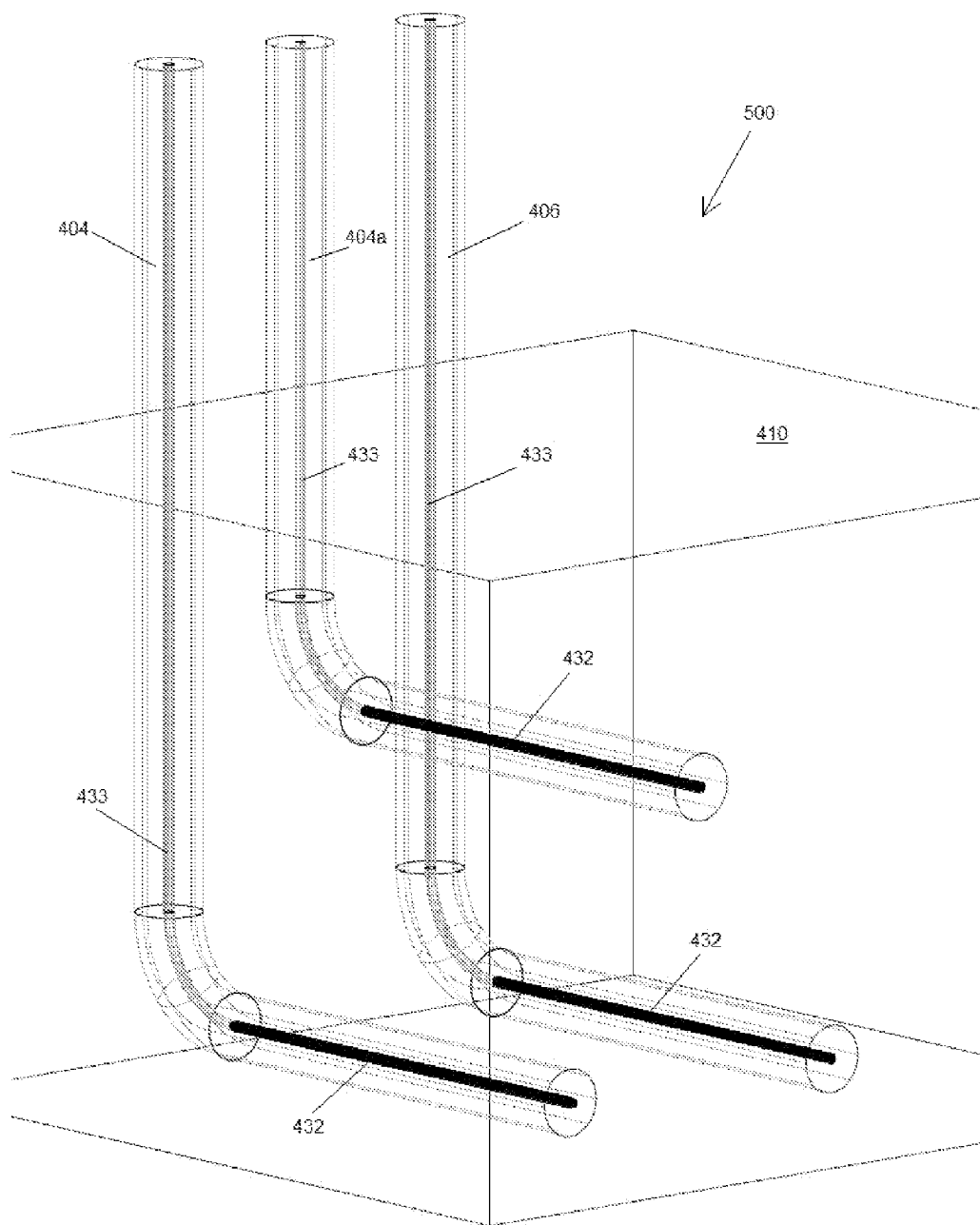
FIG. 9A
