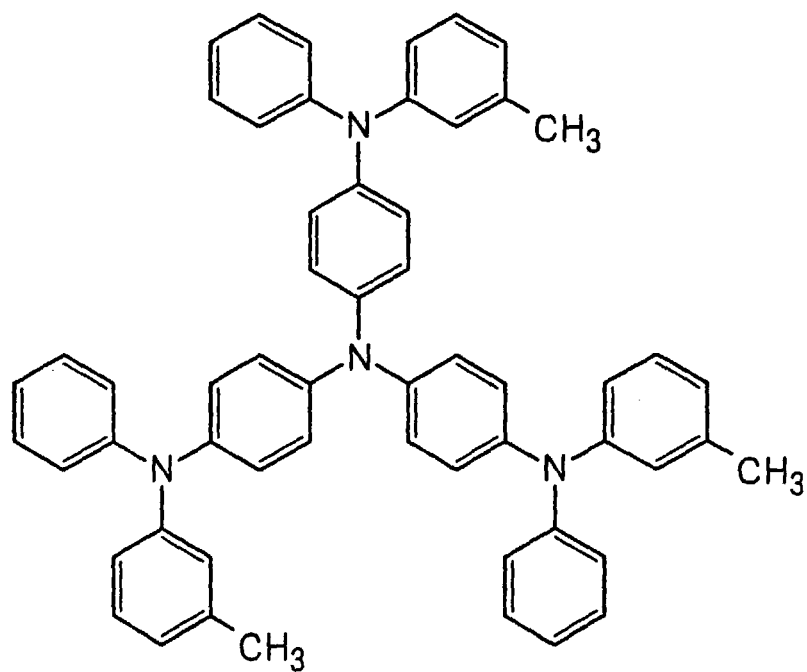
STRUCTURAL FORMULA OF m-MTDATA
