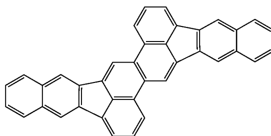
C-1
