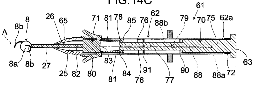
FIG. 14C
