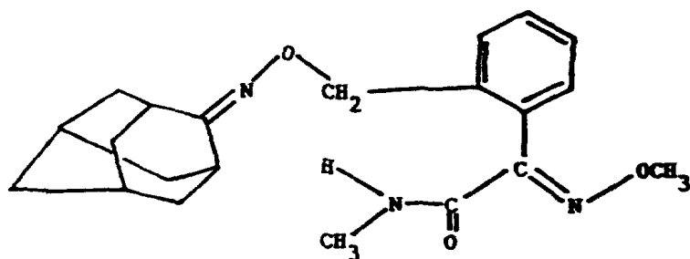
化合物318:
