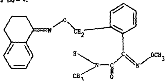
化合物55:
