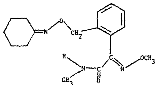
化合物54:
