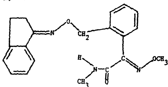
化合物152:
