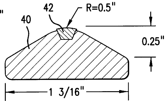
ANODE FIG. 7D
