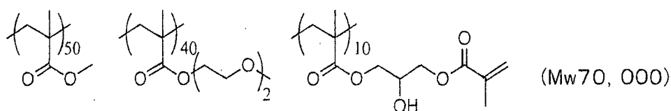
Binder polymer (1)
