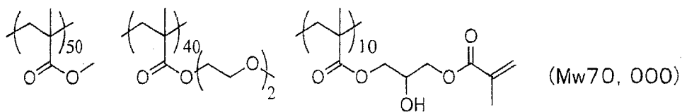
Binder polymer (1)
