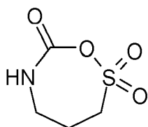
Compound D1
