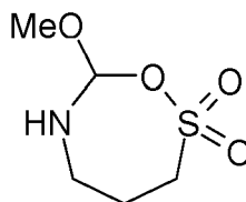
Compound D2
