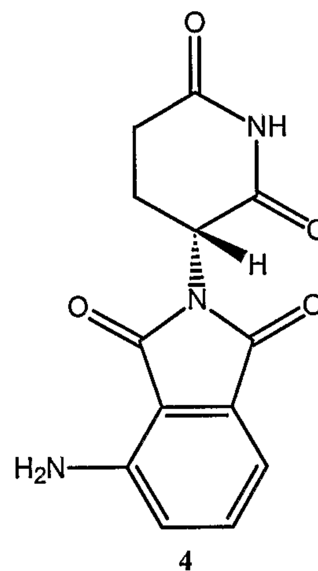
R(+)-3-amino-thalidomide
