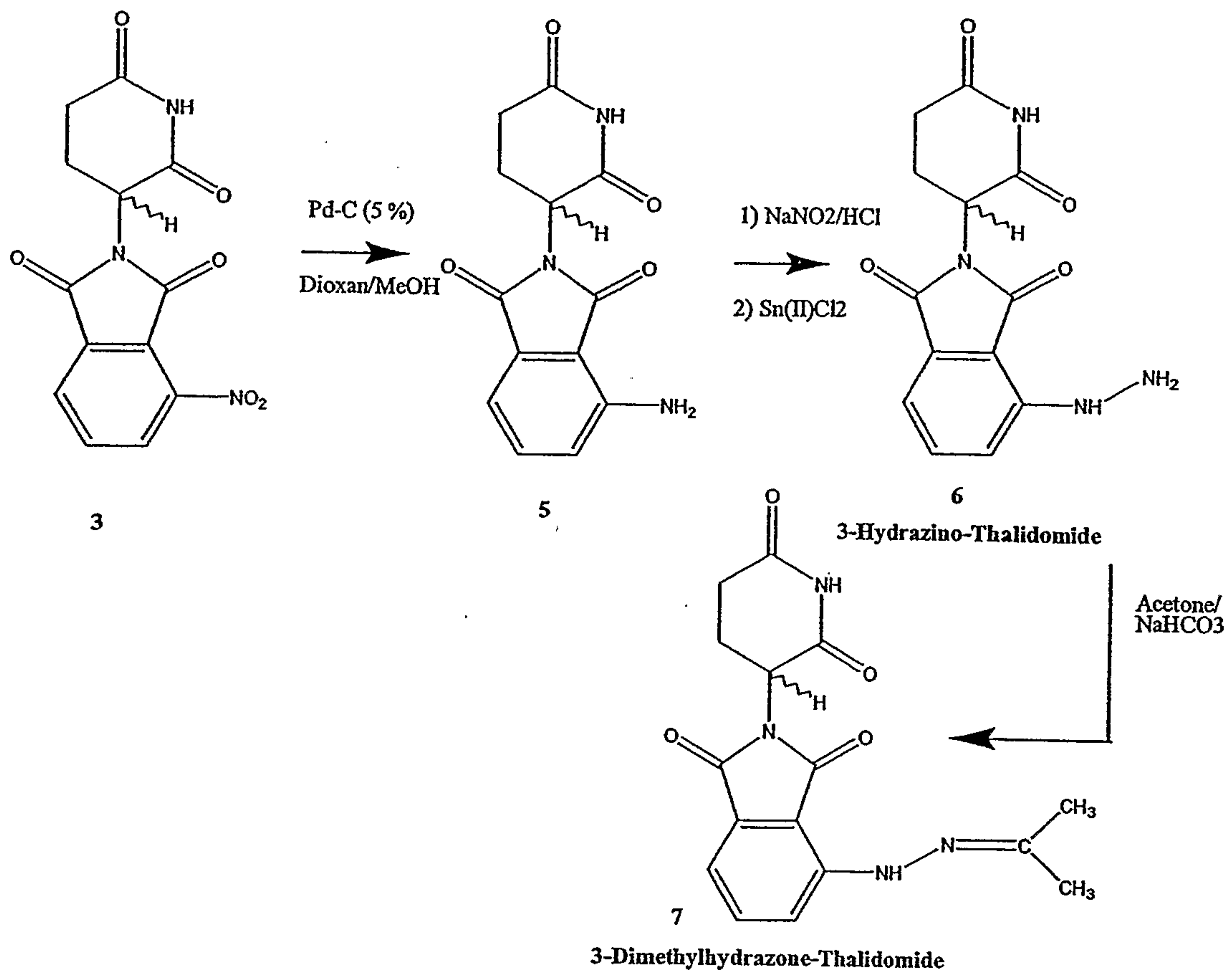
Scheme-2
