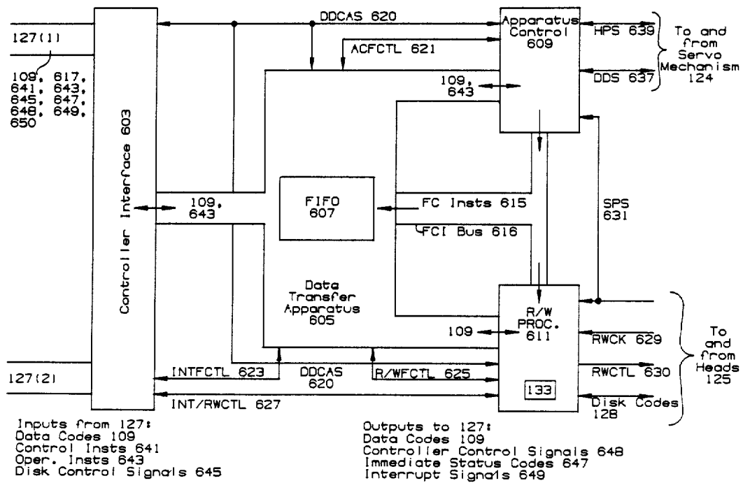
Overview of DDCA 121
