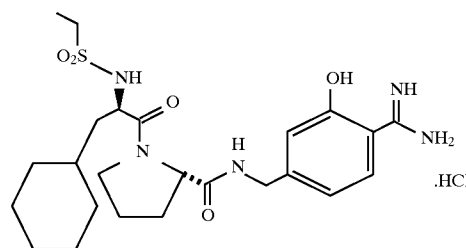
EtSO 2 -D-Cha-Pro-NHCH 2 C 6 H 3 -3-OH-4-C(NH)NH 2 .HCl
