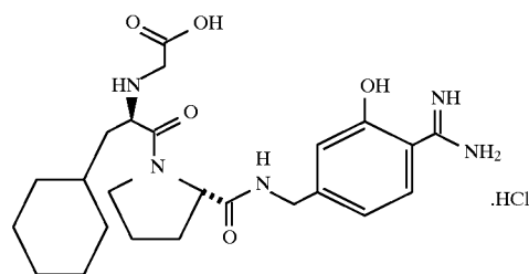
HO 2 CCH 2 -D-Cha-Pro-NHCH 2 C 6 H 3 -3-OH-4-C(NH)NH 2 .HCl
