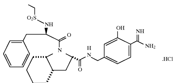
EtSO 2 -D-Phe-Ohi-NHCH 2 C 6 H 3 -3-OH-4-C(NH)NH 2 ·HCl
