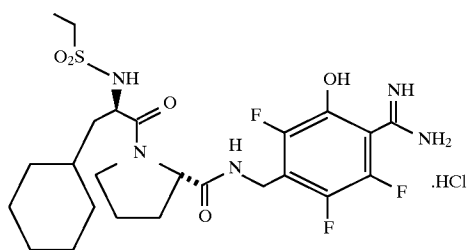
EtSO 2 -D-Cha-Pro-NHCH 2 C 6 F 3 -3-OH-4-C(NH)NH 2 ·HCl
