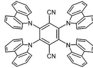
4CzTPN
