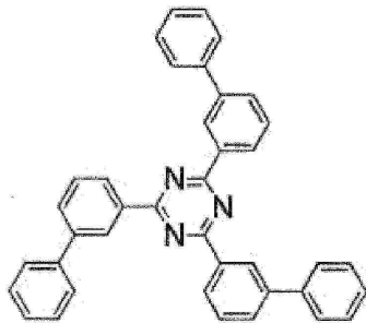
T2T
