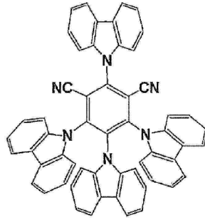
4CzIPN
