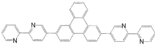
BPyTP2
