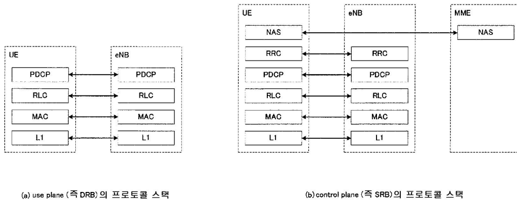
(a) use plane (즉 DRB)의 프로토콜 스택
