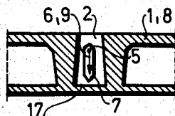
Fig. 12 K-K
