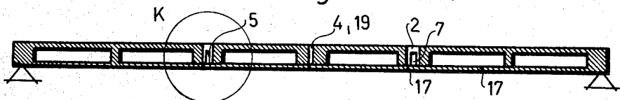
Fig. 16 I-I
