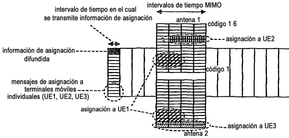
Ejemplo de información de asignación de códigos difundida en UTRA TDD
