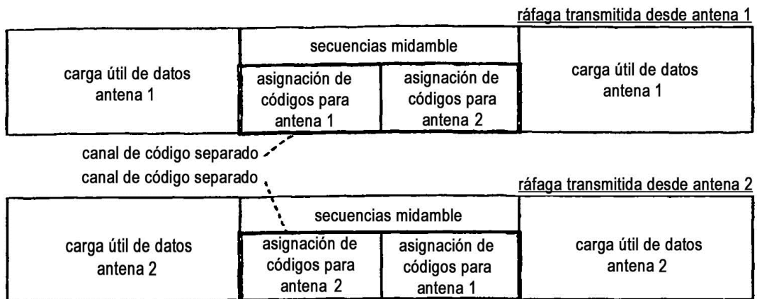
Transmisión difundida de información de asignación de códigos en parte de midamble de la ráfaga
