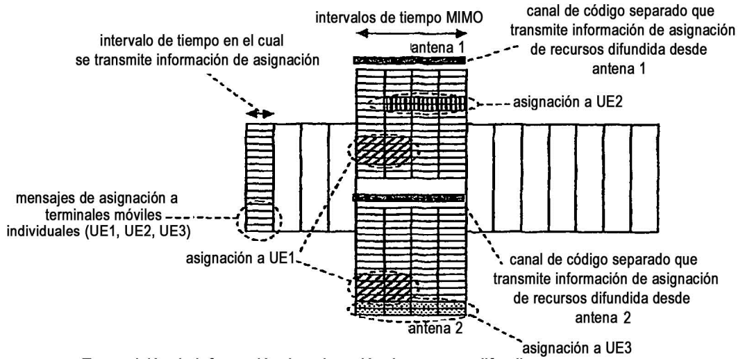
Transmisión de información de asignación de recursos difundida por medio de canal de código separado
