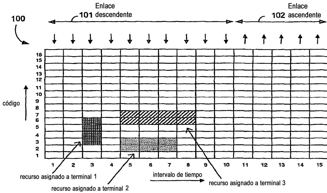
Trama de radio TDD común
