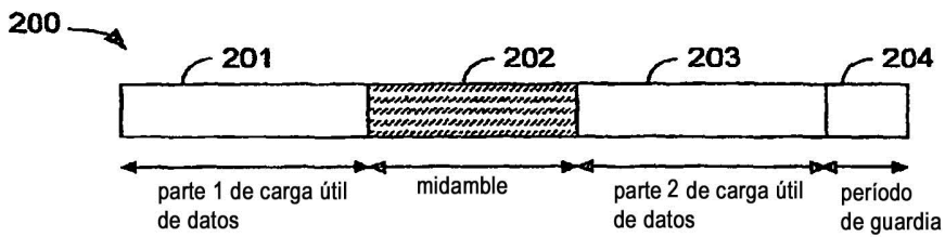
Configuración de intervalo de tiempo UTRA TDD
