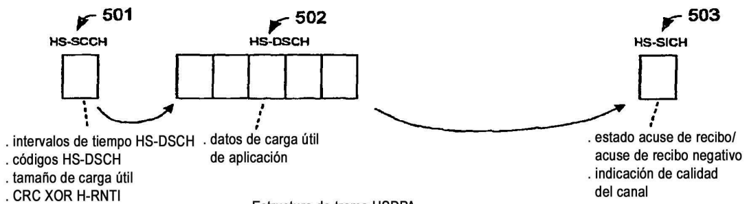
Estructura de trama HSDPA
