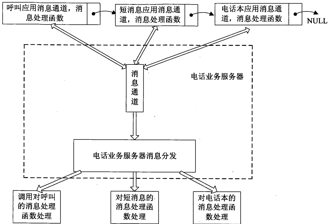
GMsgHandler对象链表
