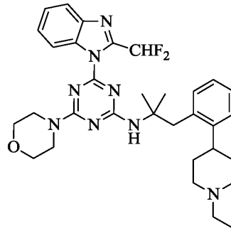
화합물 IV,
