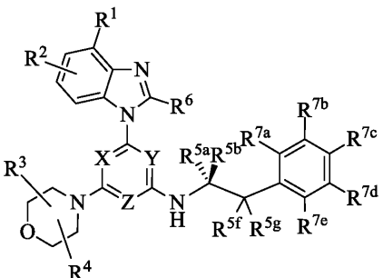
화학식 (XIb)
