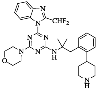
화합물 III
