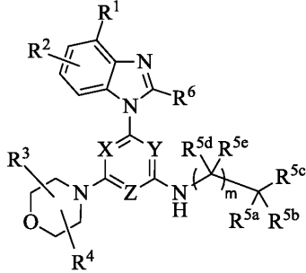
화학식 (I)
