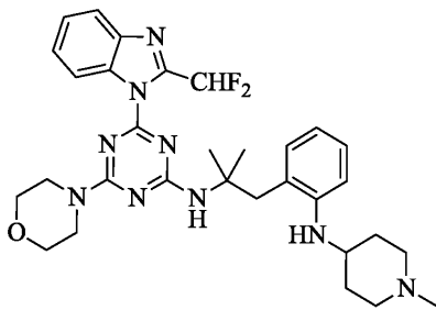
화합물 V
