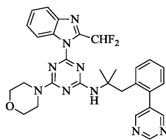
화합물 XII,
