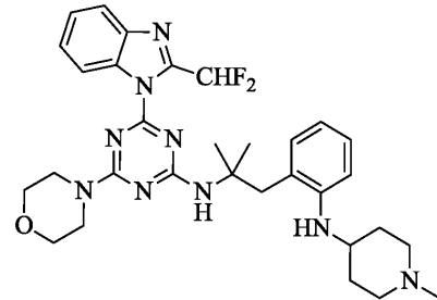
화합물 V
