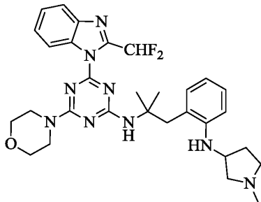
화합물 VI
