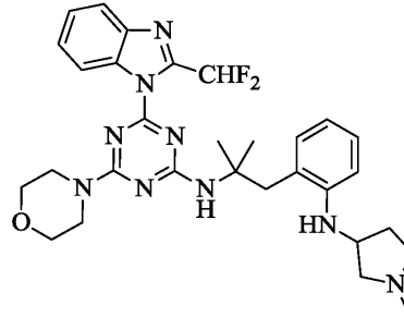
화합물 VI,
