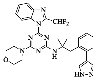
화합물 X,
