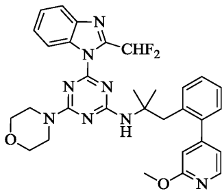
화합물 VII,
