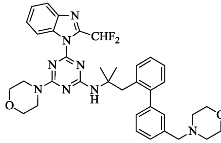
화합물 XIV,
