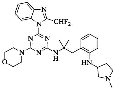
화합물 VI
