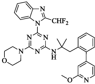
화합물 VII
