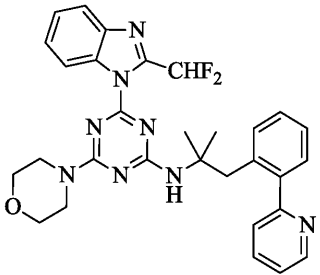
화합물 VIII
