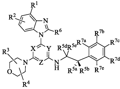
화학식 (IXb)
