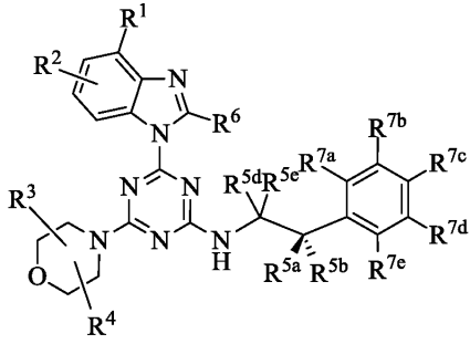
화학식 (Xa)
