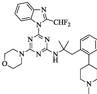
화합물 I
