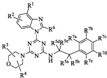
화학식 (X)
