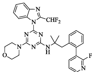
화합물 XI,
