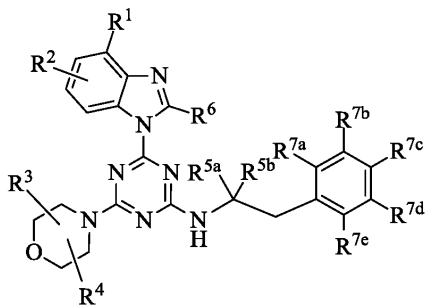
화학식 (XVI)
