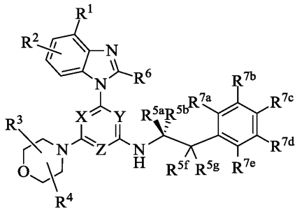
화학식 (XIa)
