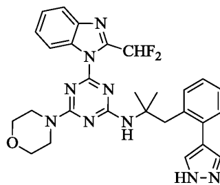
화합물 X
