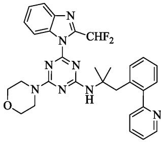
화합물 VIII
