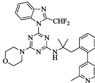
화합물 IX
