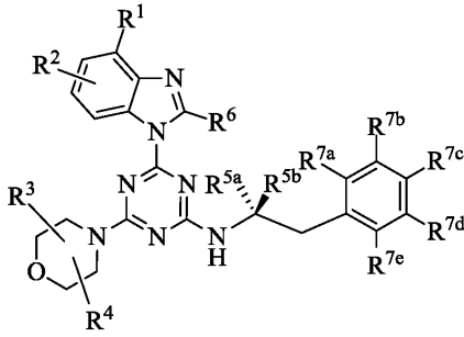
화학식 (XVIIb)
