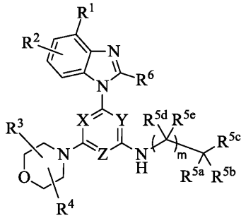
화학식 (I)
