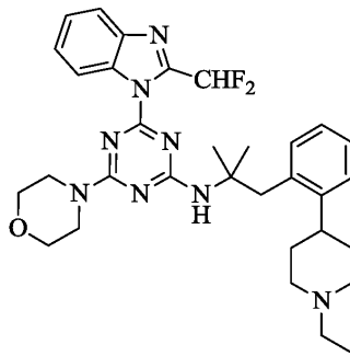
화합물 IV
