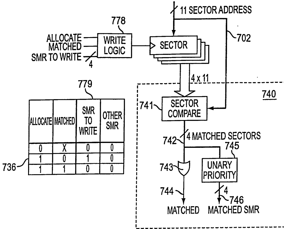
Sector match logic FIG. 7E
