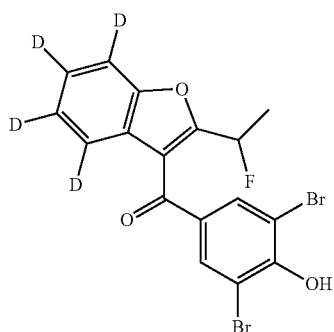
2,6-dibromo-4-[2-(1-fluoroethyl)( 2 H 4 )-1-benzofuran-3-carbonyl]phenol
