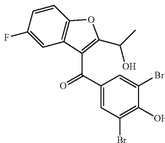
2,6-dibromo-4-[5-fluoro-2-(1-hydroxyethyl)-1-benzofuran-3-carbonyl]phenol
