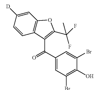
2,6-dibromo-4-[2-(1,1-difluoroethyl)(6- 2 H)-1-benzofuran-3-carbonyl]phenol
