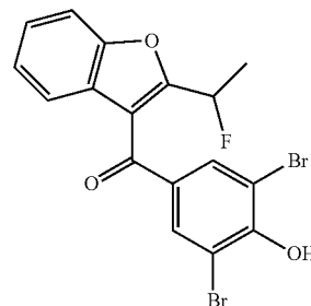
2,6-dibromo-4-[2-(1-fluoroethyl)-1-benzofuran-3-carbonyl]phenol
