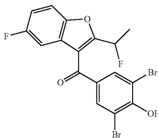
2,6-dibromo-4-[5-fluoro-2-(1-fluoroethyl)-1-benzofuran-3-carbonyl]phenol
