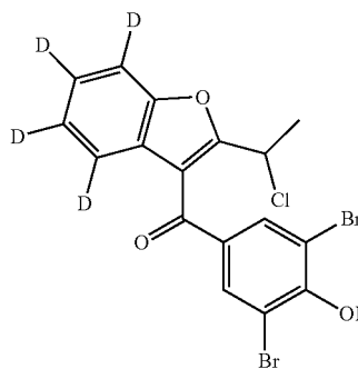
2,6-dibromo-4-[2-(1-chloroethyl)( 2 H 4 )-1-benzofuran-3-carbonyl]phenol
