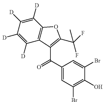
2,6-dibromo-4-[2-(1,1-difluoroethyl)( 2 H 4 )-1-benzofuran-3-carbonyl]phenol
