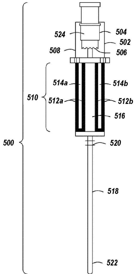
FIG. 5A
