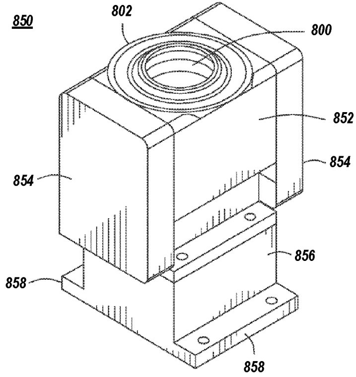
FIG. 8C
