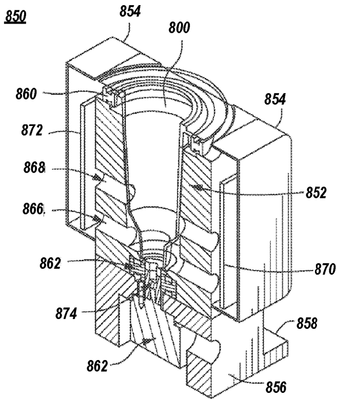
FIG. 8D
