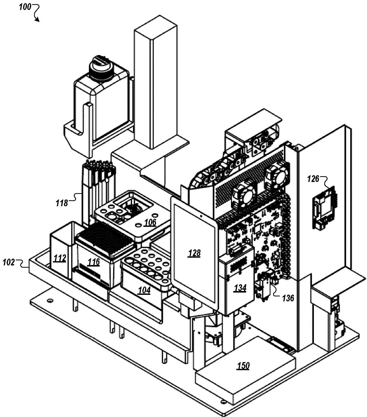
FIG. 1B
