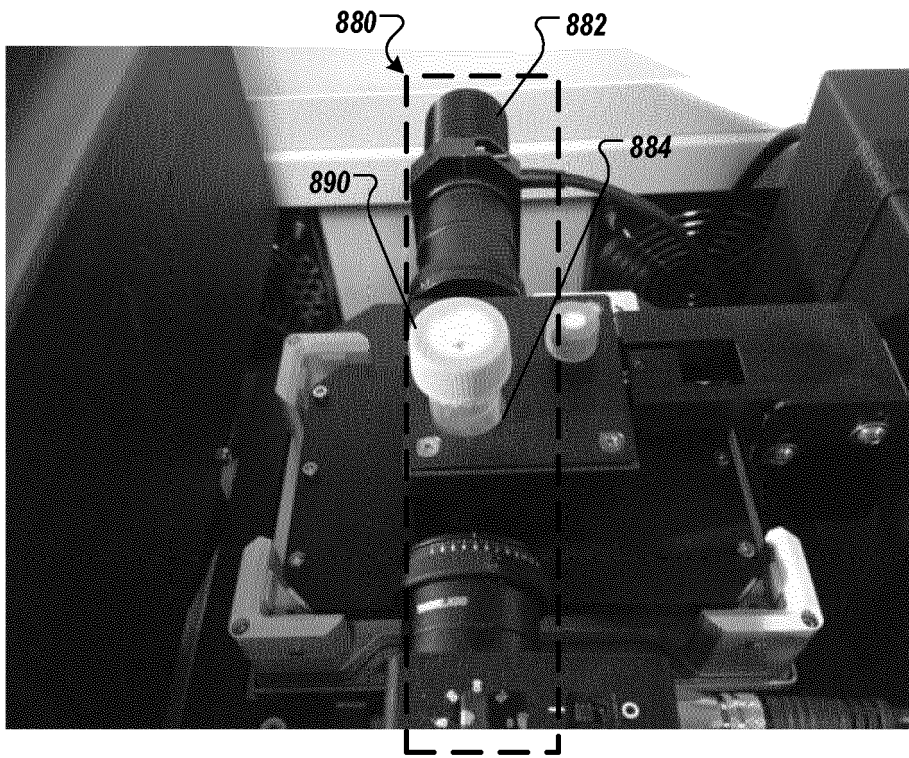
FIG. 8E
