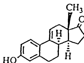
\Delta 9(11) -désydro-8-isoestrone (VI)
