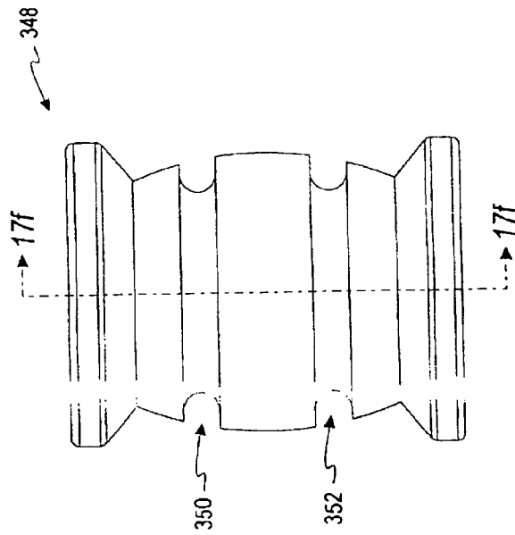
FIG. 17e
