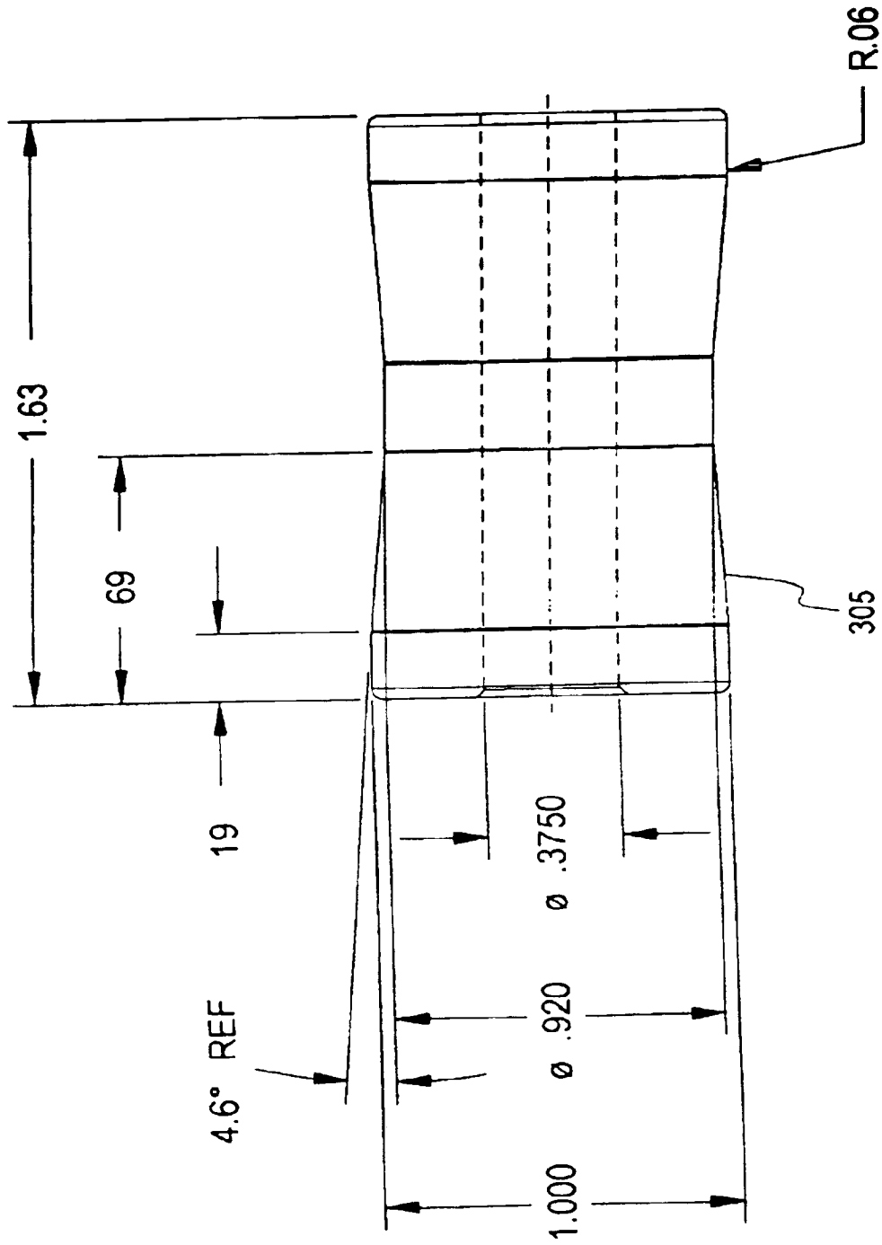
FIG. 17d
