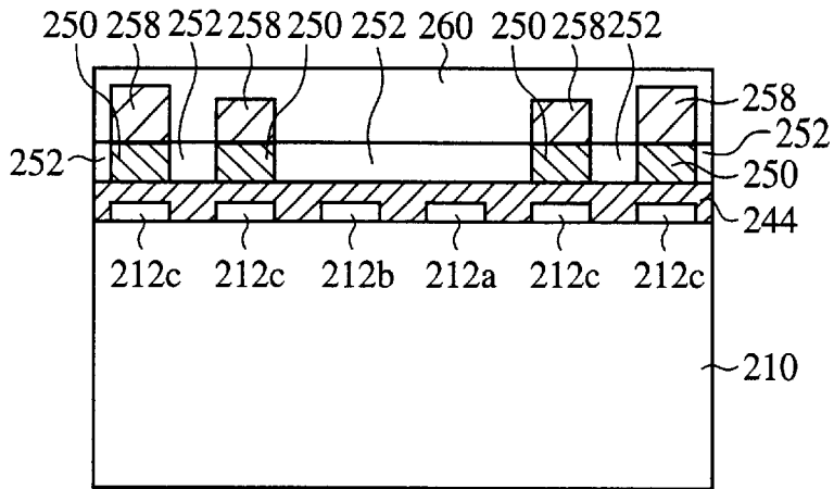
FIG. 21C
