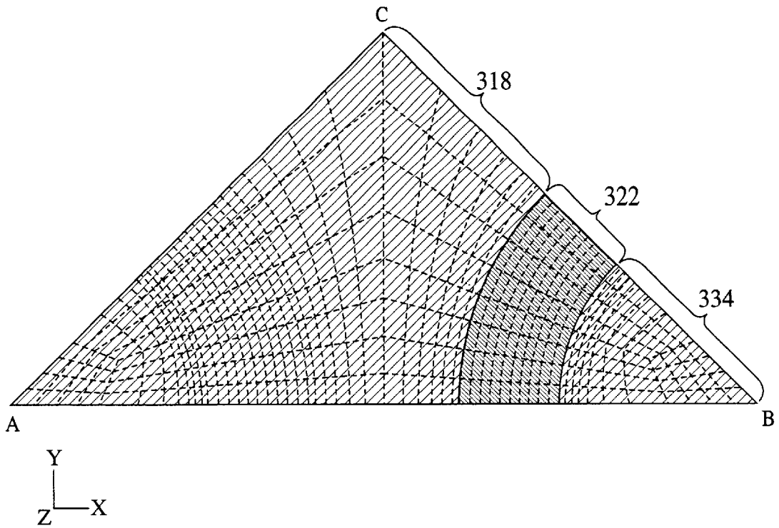
FIG. 37B
