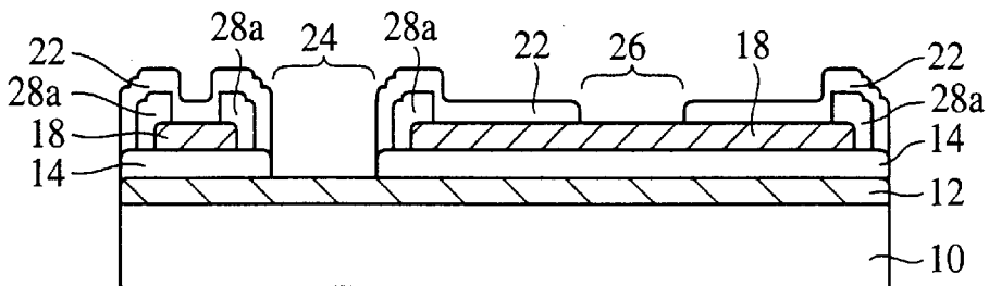
FIG. 8D
