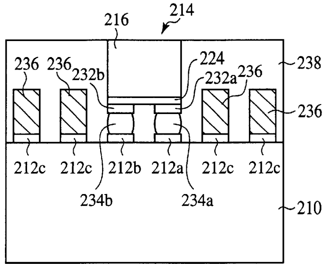
FIG. 23B
