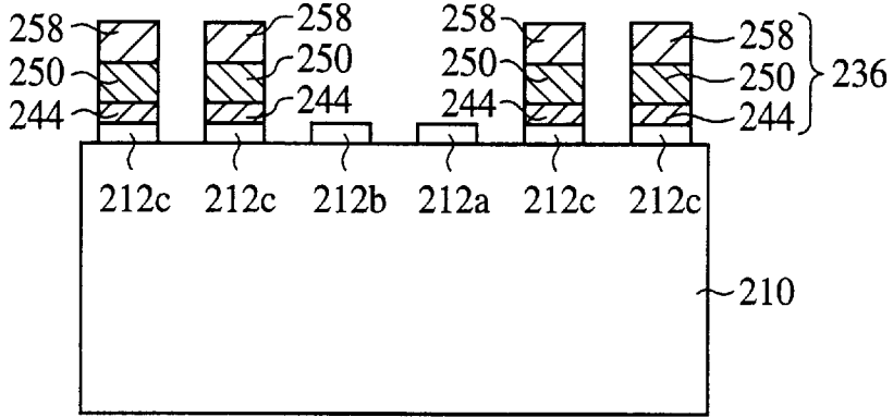
FIG. 22B
