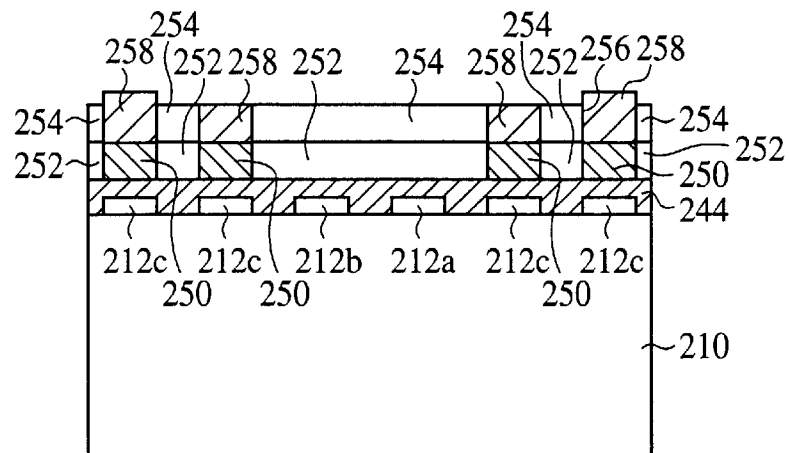
FIG. 20C
