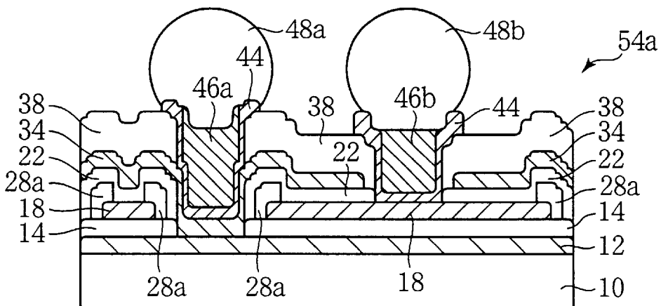
FIG. 10C
