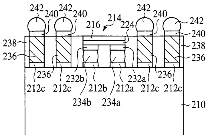
FIG. 23C
