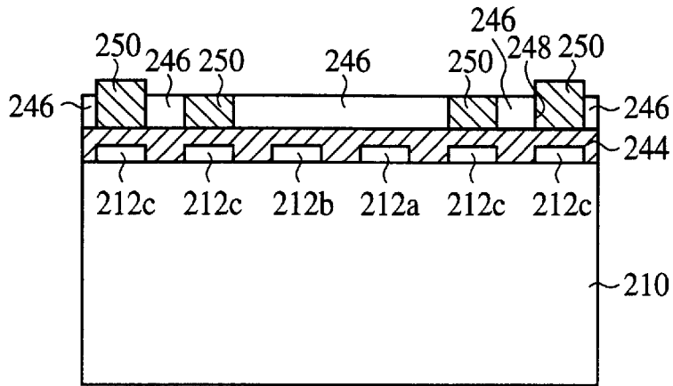
FIG. 19A
