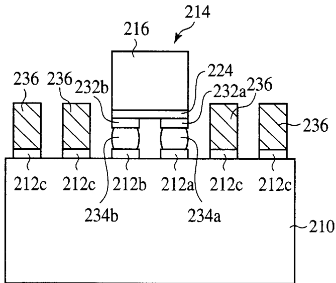
FIG. 22C
