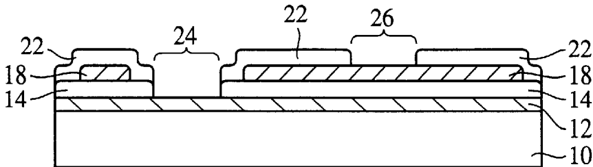
FIG. 3C
