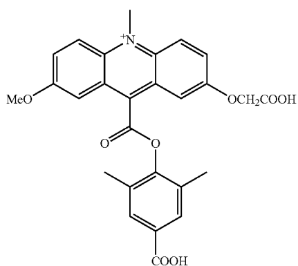
2-CME-7-methoxy-DMAE
