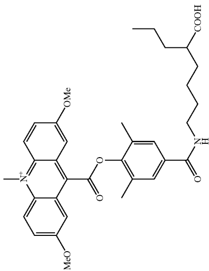
2,7-dimethoxy-DMAE-valproate
