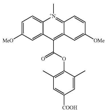
2,7-dimethoxy-DMAE
