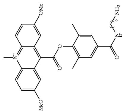
2,7-dimethoxy-DMAE-HD
