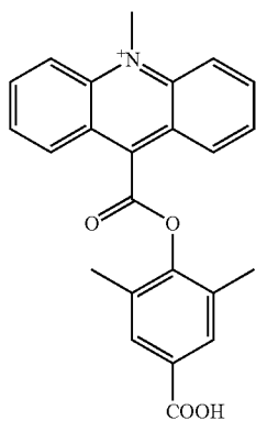
DMAE
