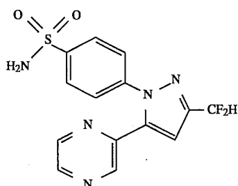
4-[5-(4-Pyrazinyl)-3-(difluoromethyl)-1H-pyrazol-1-yl]benzenesulfonamide
