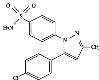
4-[5-(4-Chlorophenyl)-3-trifluoromethyl]-1H-pyrazolyl]benzenesulfonamide
