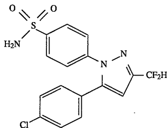
4-[5-(4-Chlorophenyl)-3-(difluoromethyl)-1H-pyrazol-1-yl]benzenesulfonamide
