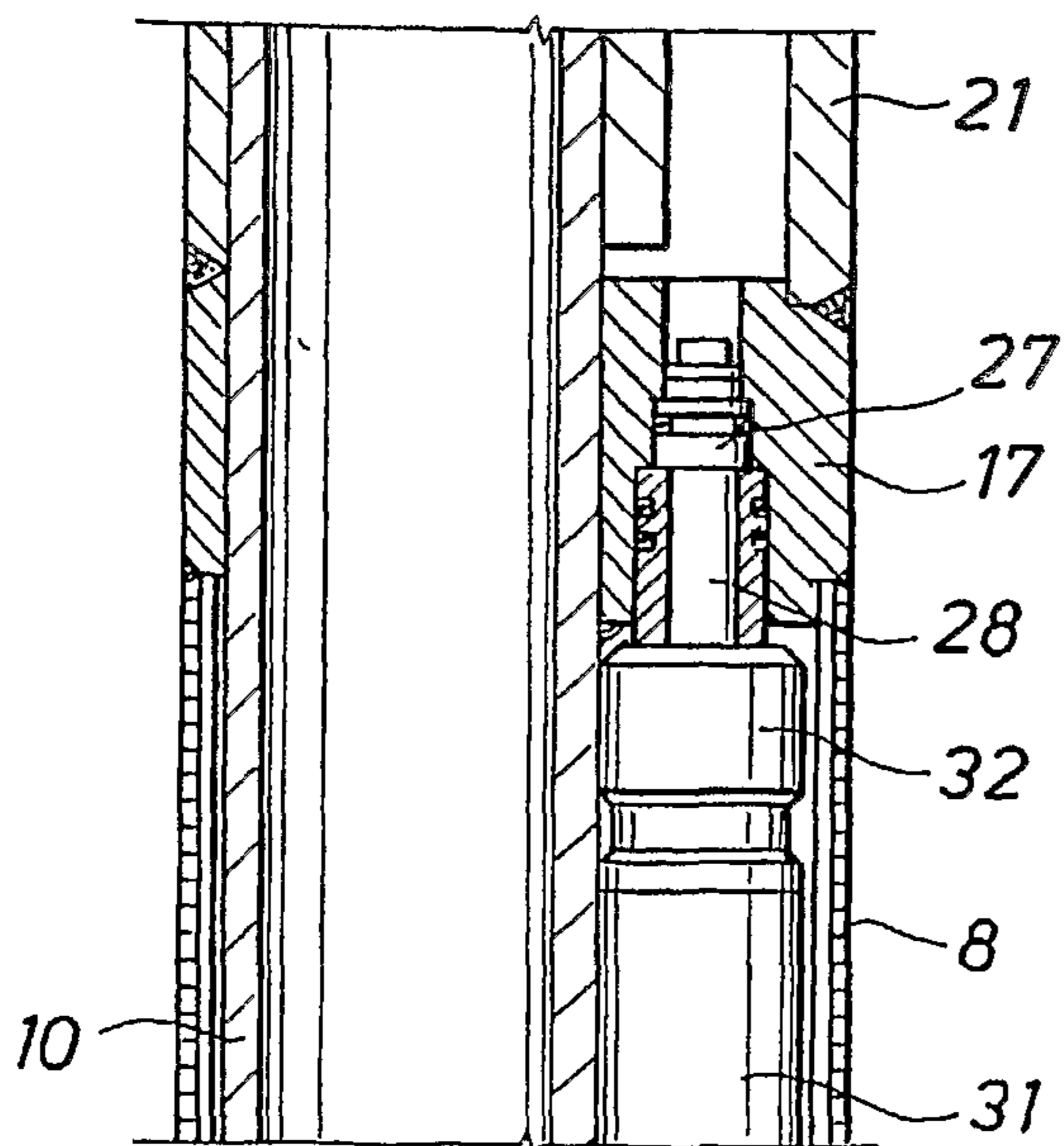
FIG. 5C
