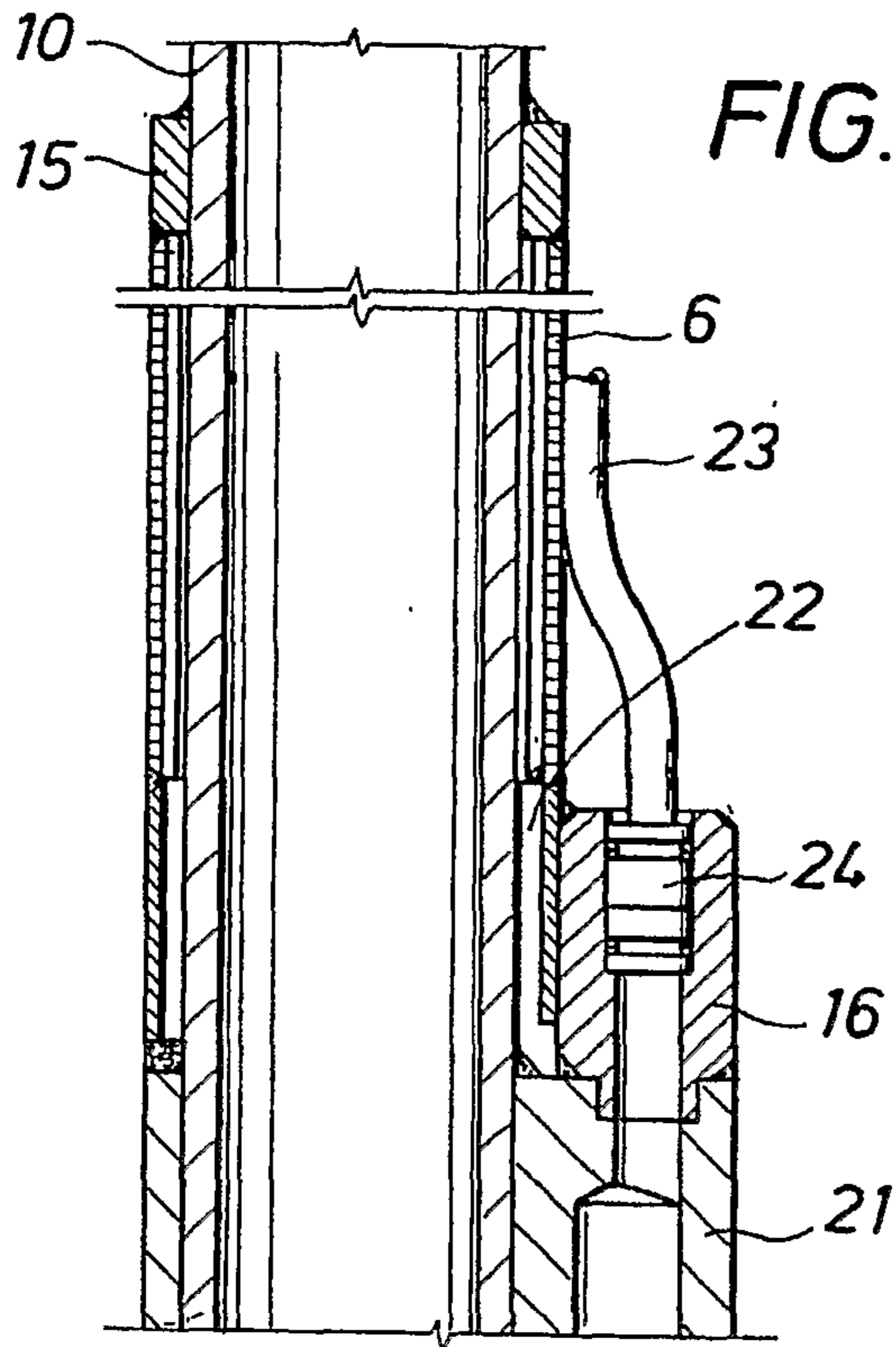
FIG. 5B
