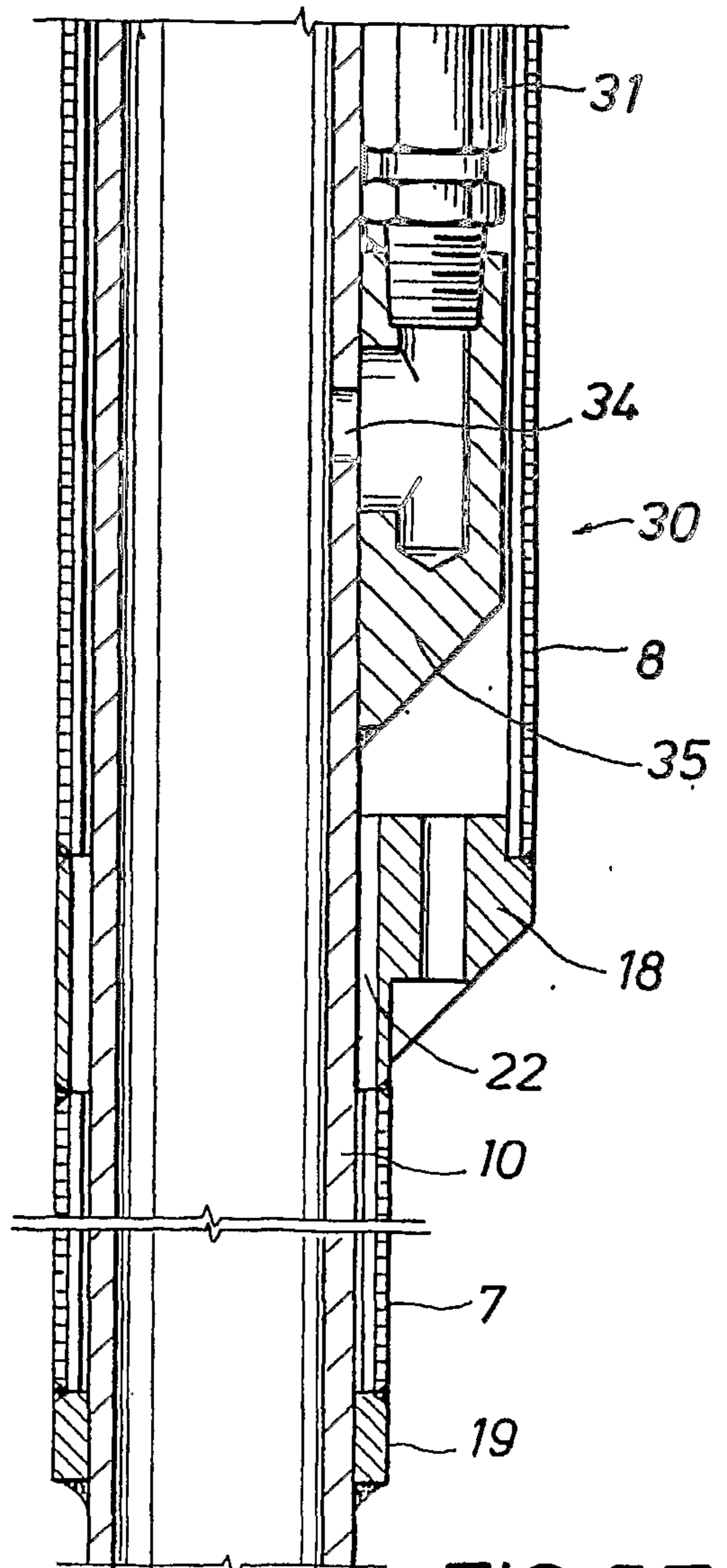
FIG. 5E
