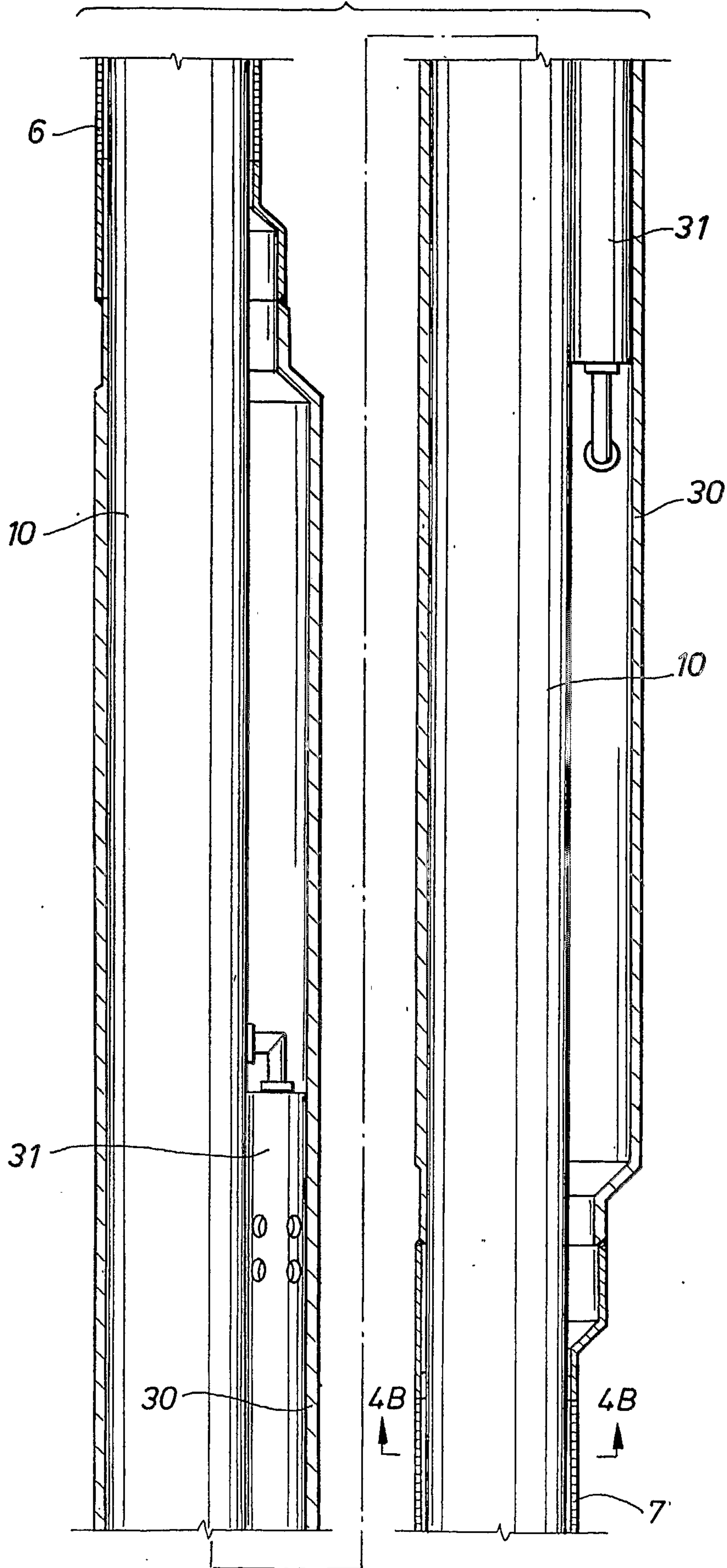
3/12 FIG. 4A
