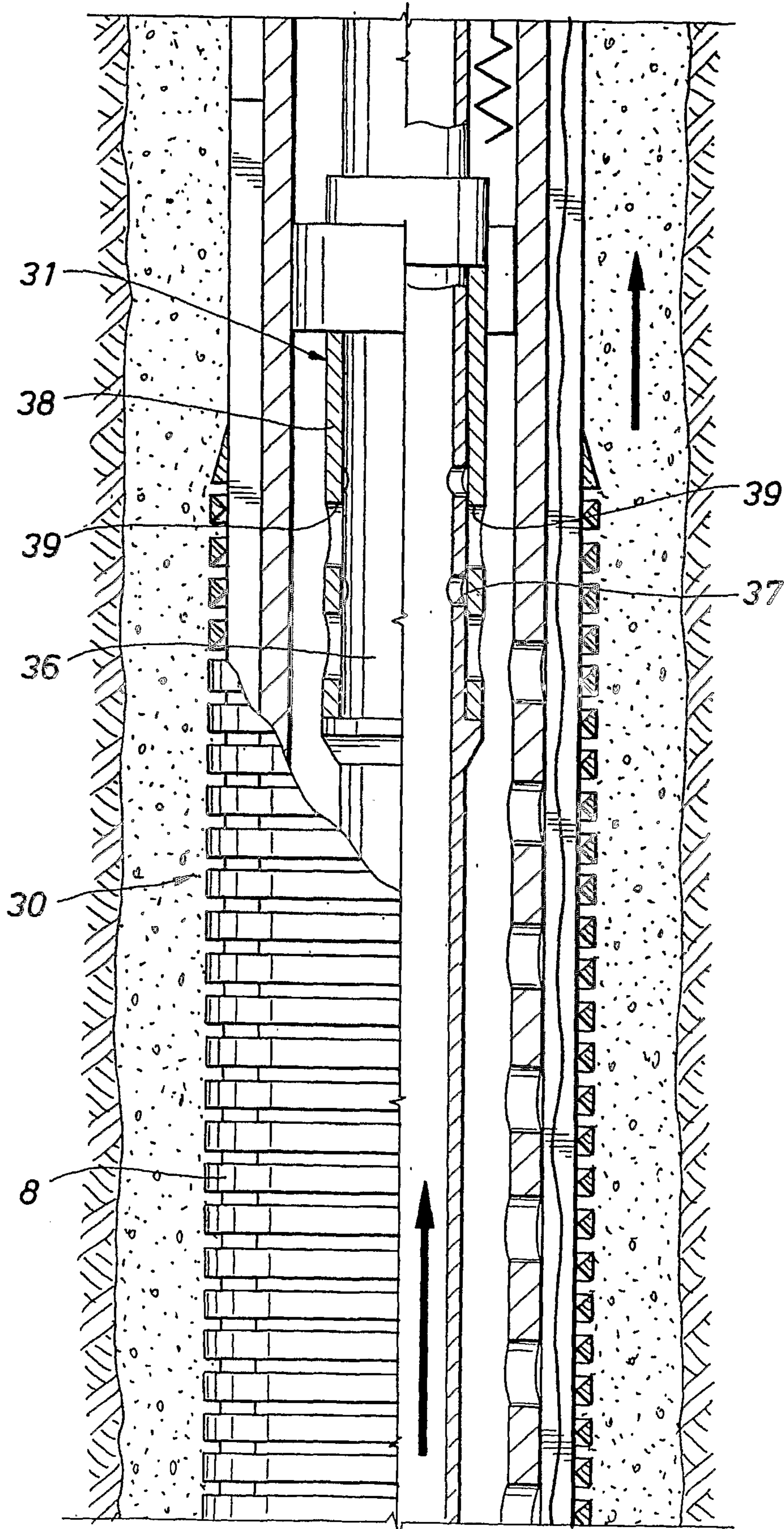
FIG. 11
