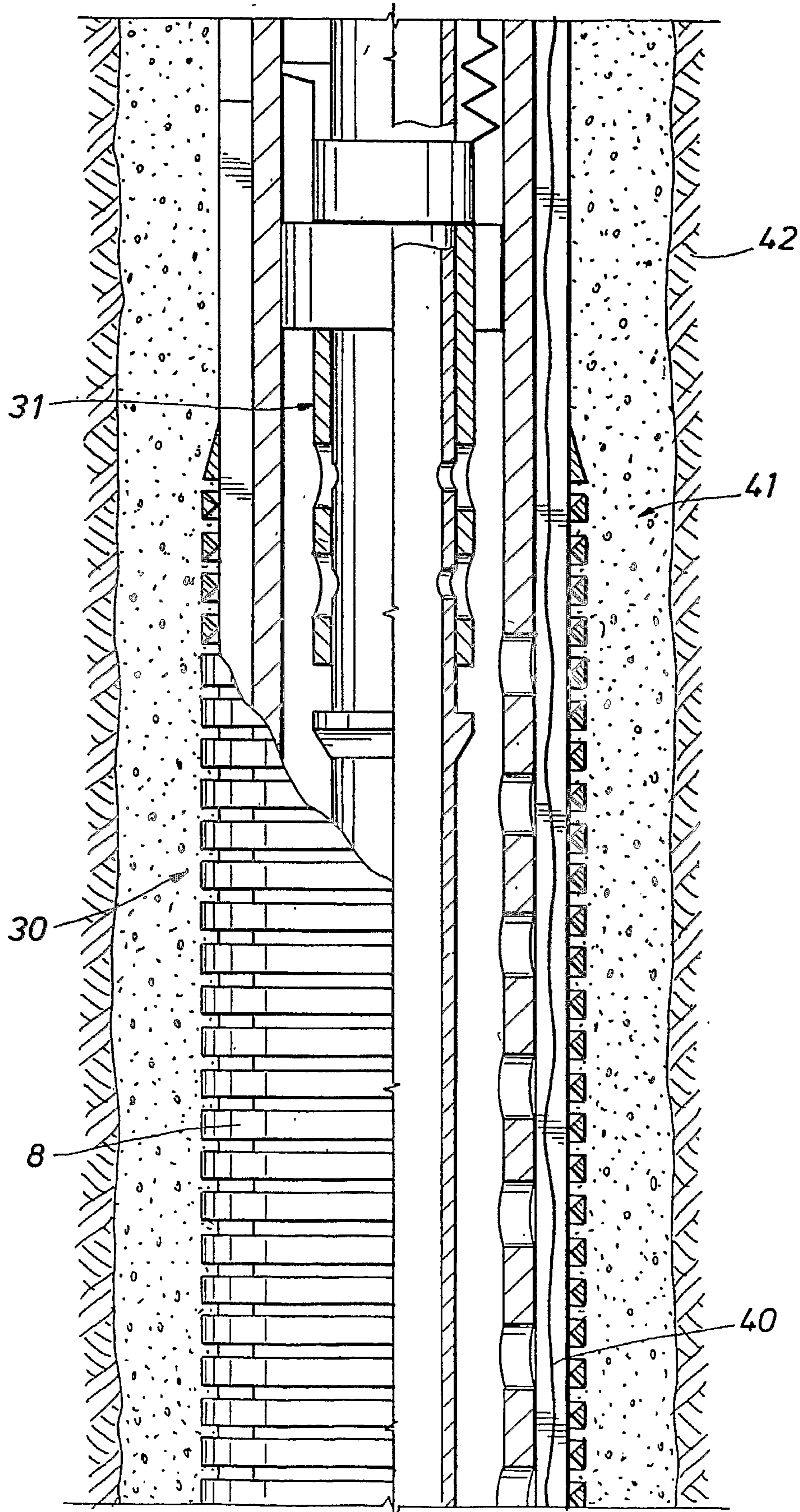
FIG. 9
