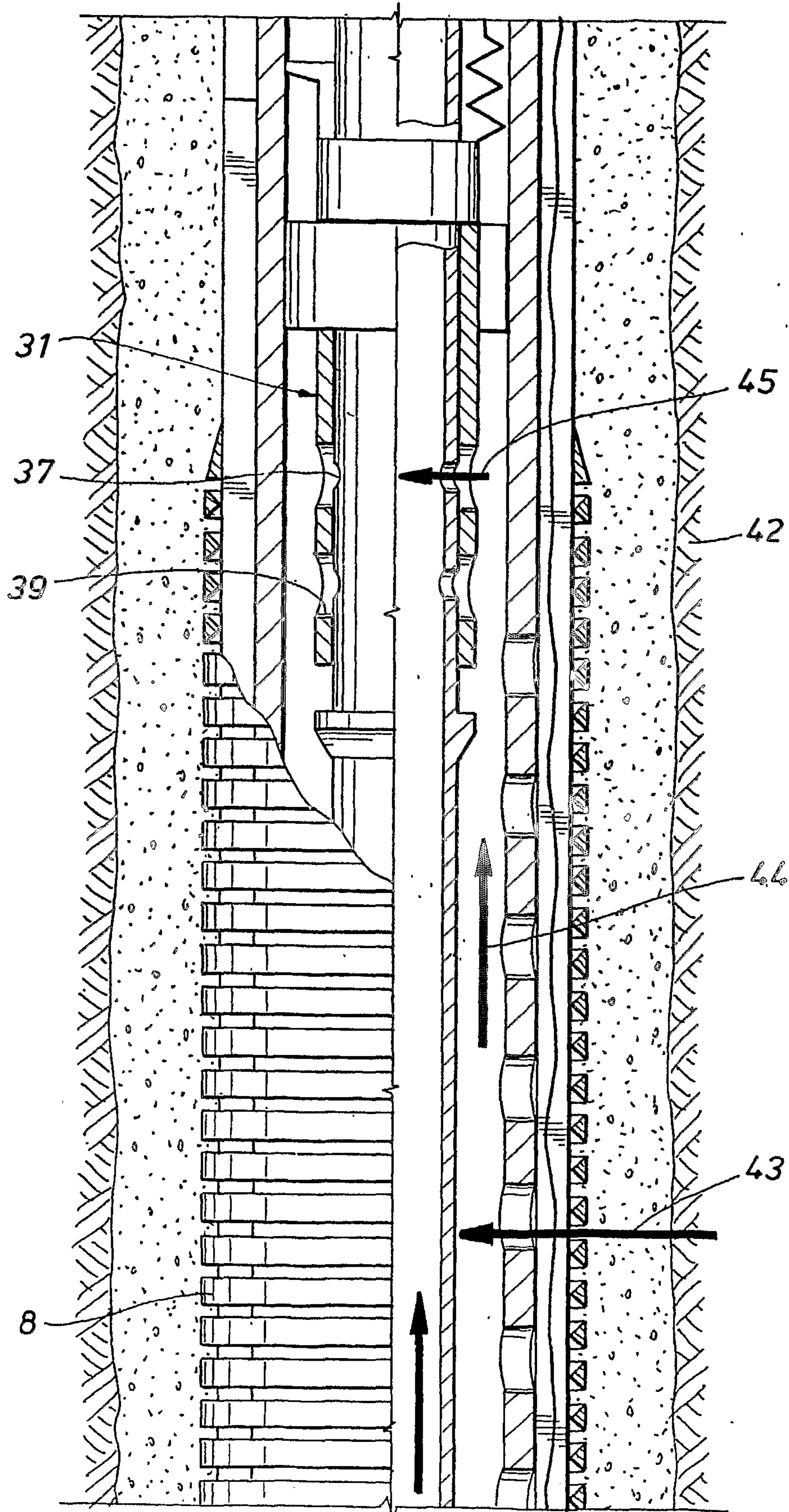
FIG. 10
