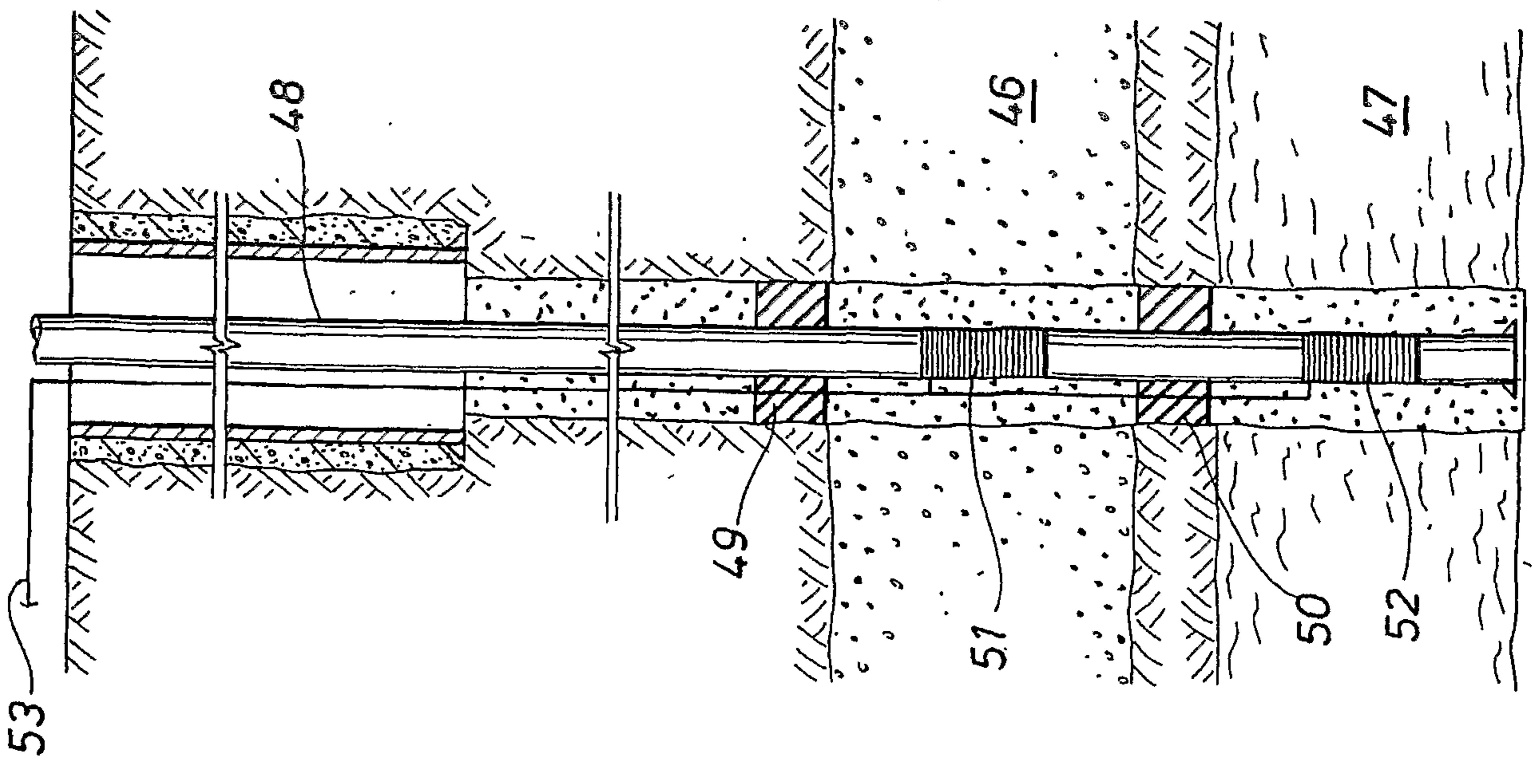
FIG. 12
