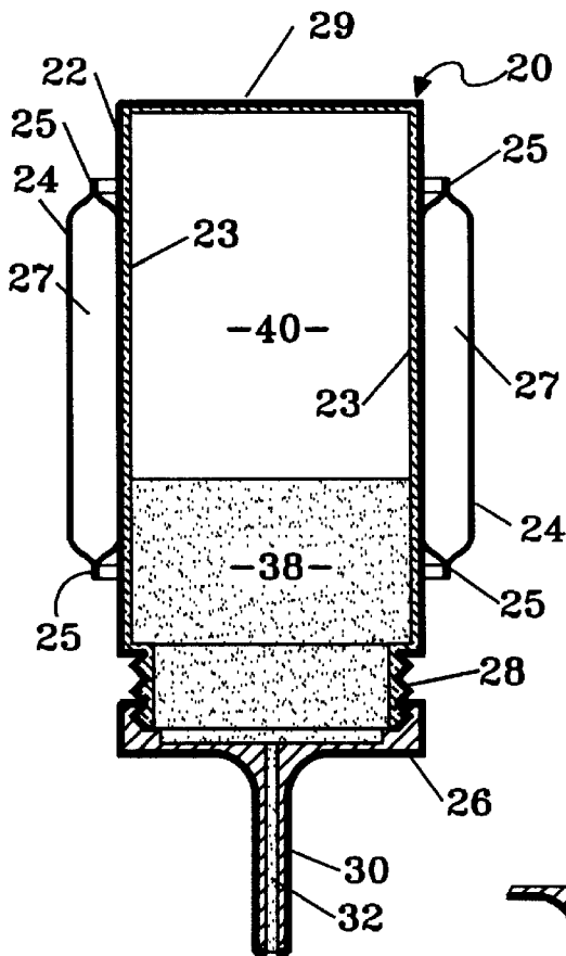
Fig. 2A SECTION A:A
