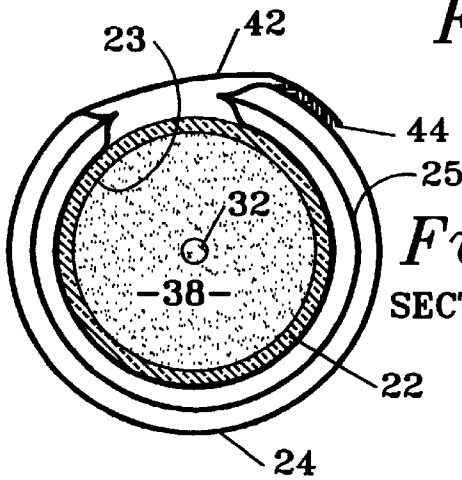
Fig. 2A SECTION A:A
