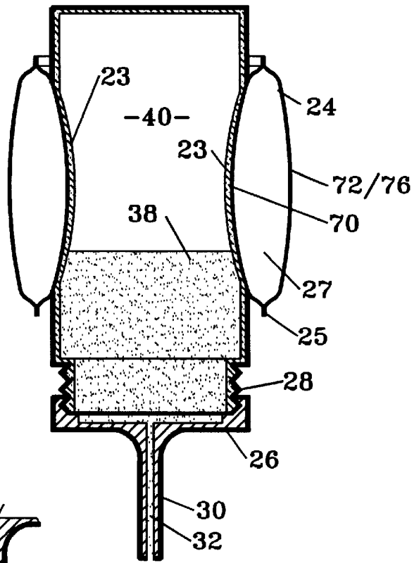
Fig. 2B SECTION A:A
