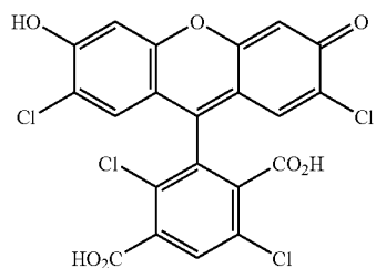
TET
