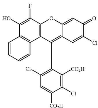
Cl-FLAN
