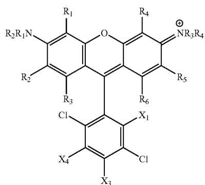
4,7-Dichlororhodamine
