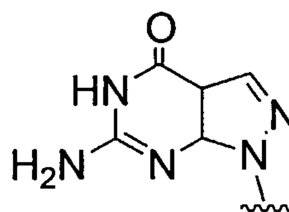
N9-(7-deaza-8-aza-Guanine)
