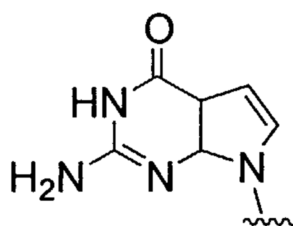
N9-(7-deaza-Guanine)
