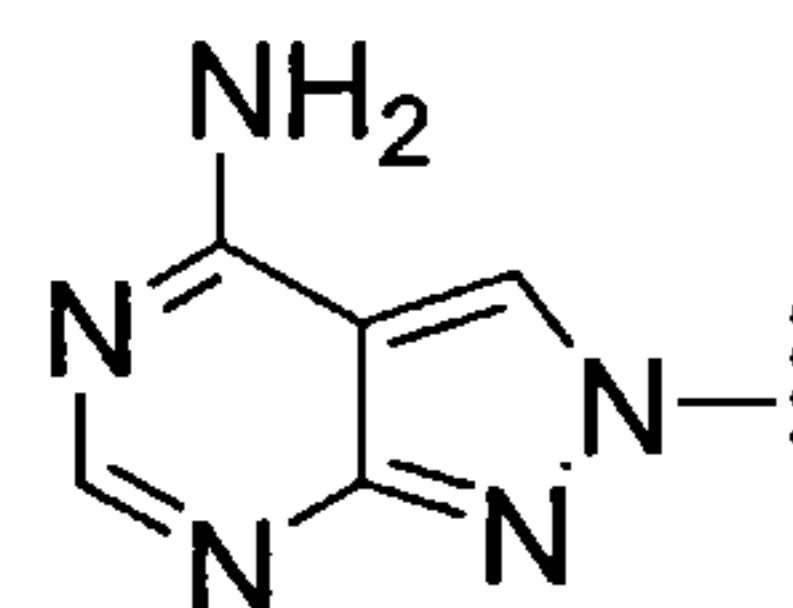
N8-(7-deaza-8-aza-Adenine)
