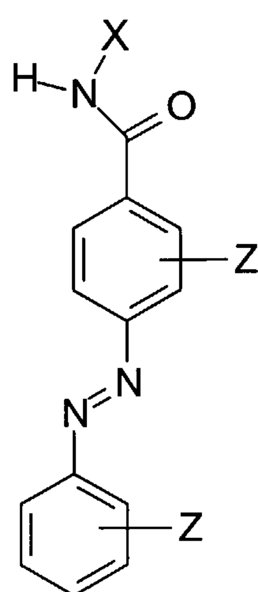
Dabcy1
